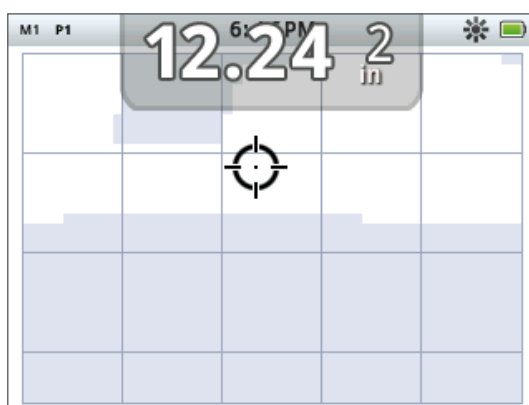
Figure 8 – Ecran Détecter affichant l'échelle de discrimination
