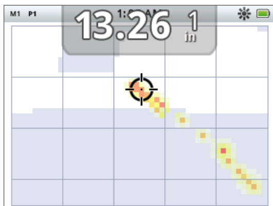
Figure 12 – Trace cible affichant deux cibles (monnaie et clou)
