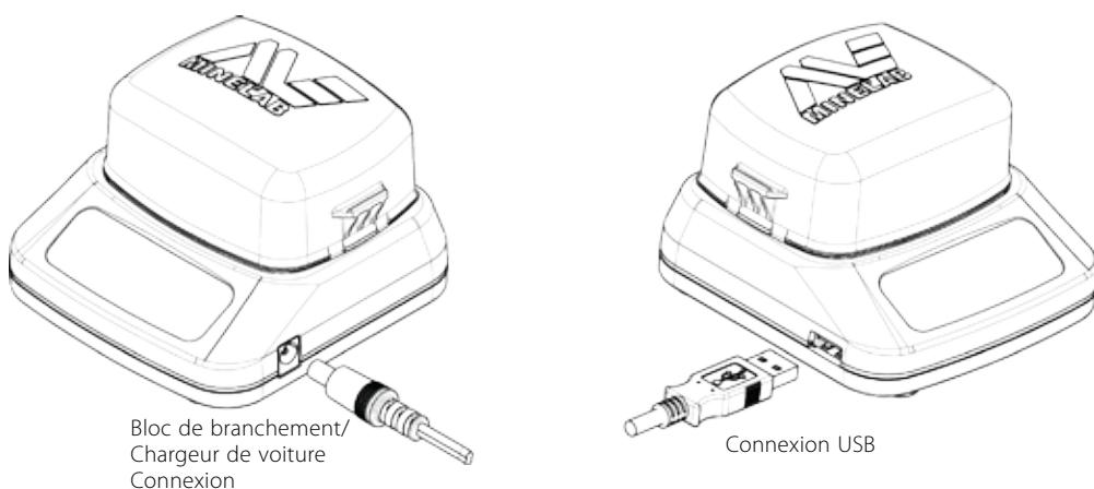
Figure 36 – Connexions du connecteur d'alimentation du BC 10 et USB
