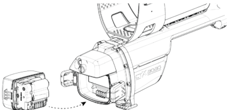
Figure 40 – Remplacez les piles AA
