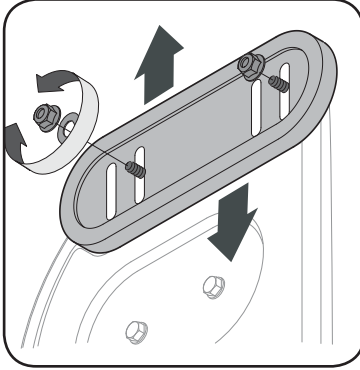
Figure 5-8-Patins réversibles en plastique
