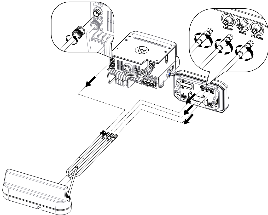
Abbildung 6: Lösen der Kabel (MXM7000 mit 2-DIN-Konfiguration)
