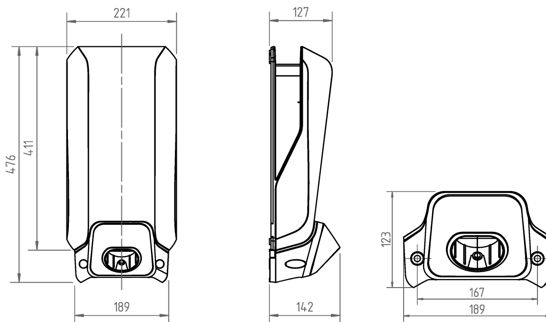
Abb. 22-5: Abmessungen in Millimeter
