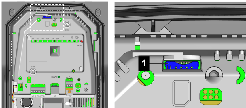
1 ... SIM-Kartensteckplatz
