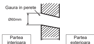
Secțiunea gaurii din perete © Teava gaurii de conducta
