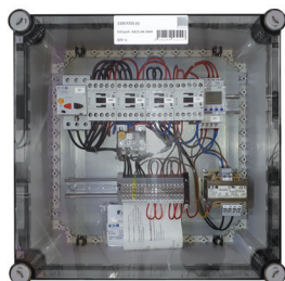
Coffret de désenfumage parking habitat collectif
