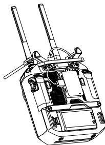
将天线穿入天线夹，注意安装时天线应位于槽内，切勿压到，否则容易损坏天线。
