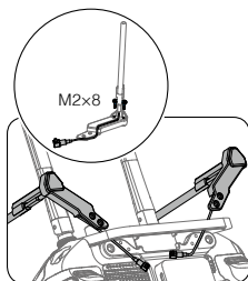
將天線穿入天線夾中，注意安裝時天線應位於槽內，切勿壓到，否則容易損壞天線。
