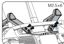
使用螺丝固定天线夹到挂载板上，最后连接天线到天空端。
