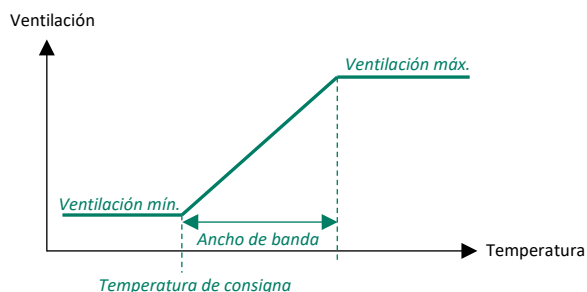
Fig. 1: Gráfico de ancho de banda
