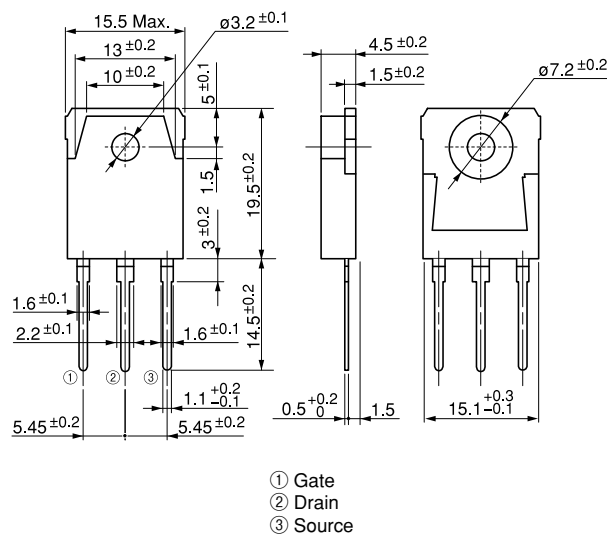
TO-3P(Q)
