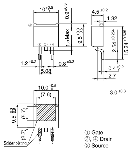
T-Pack(SJ) [D2-Pack]
