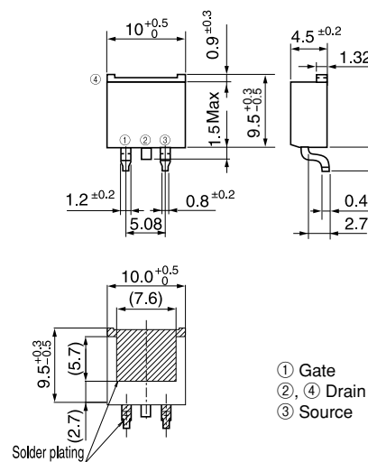
T-Pack(S)
