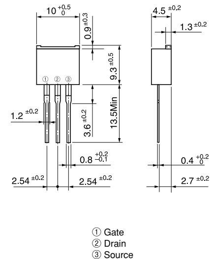
T-Pack(L)
