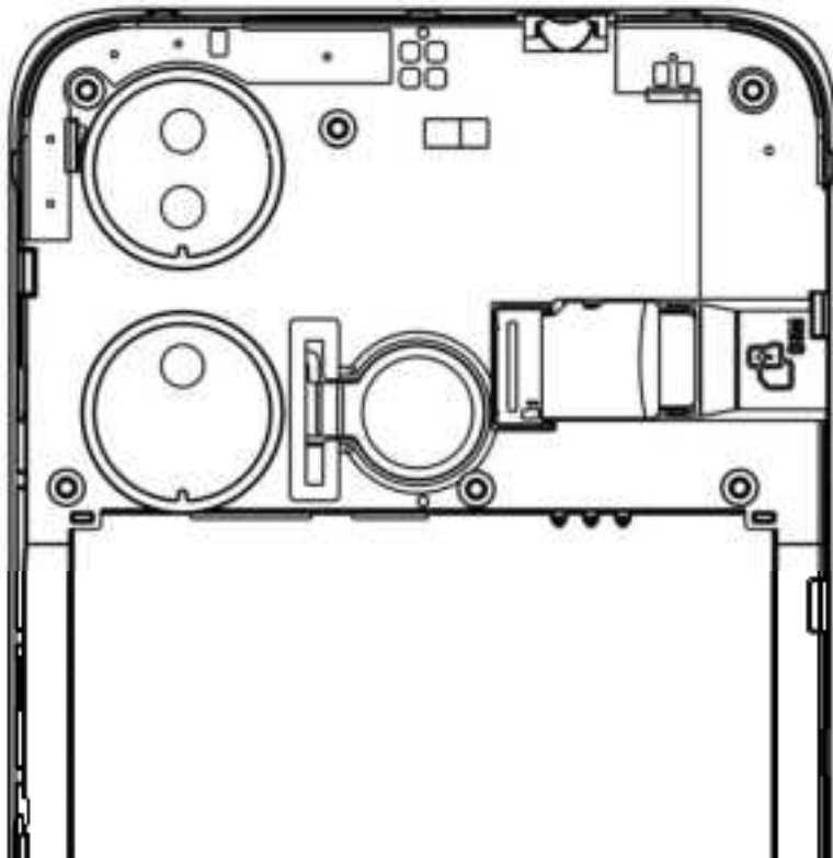
Slot para cartão SIM
