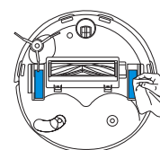
Roues motrices
