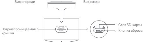
Вид сзади
