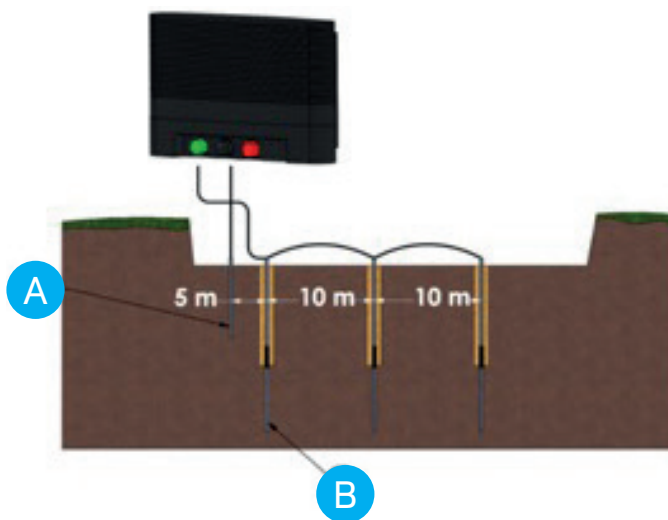
Figur 3.2: Exempel jordningsmodell MBS3000i
