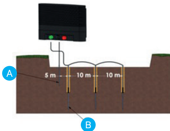
Figur 3.2: Erdung Beispiel Model MBS3000i
