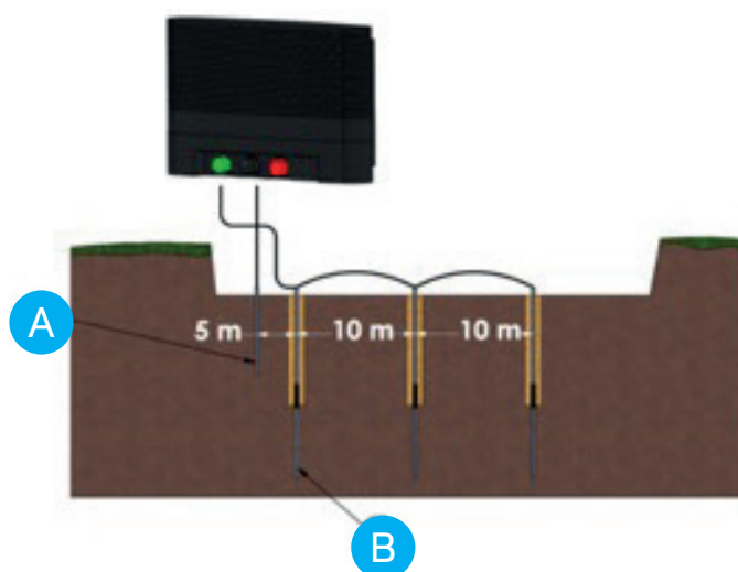
Figur 3.2: Eksempel jordforbindelsesmodel MBS3000i
