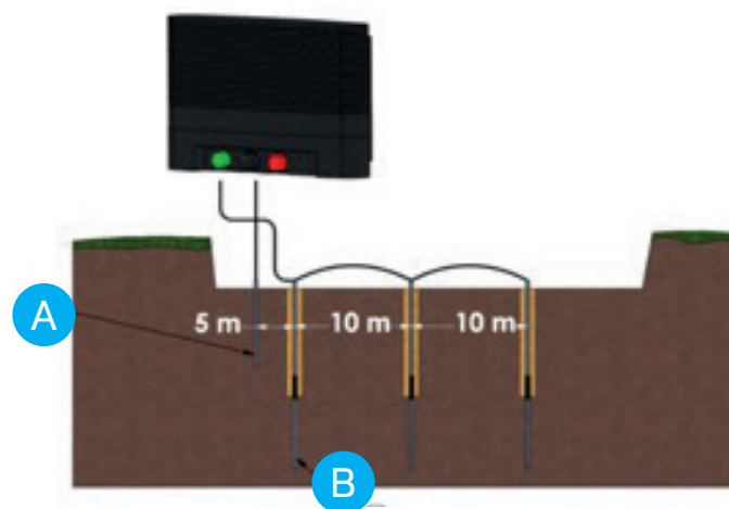
Illustration 3.2 : Schéma de mise à la terre du MBS3000i
