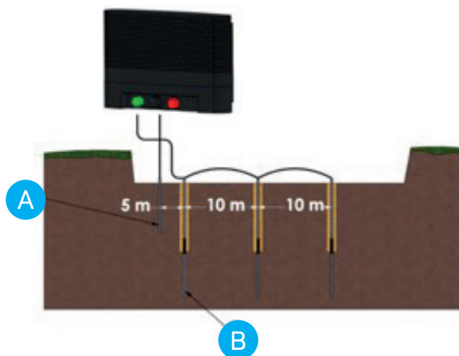
Afb. 3.2: Aarding schema voor type MBS3000i.
