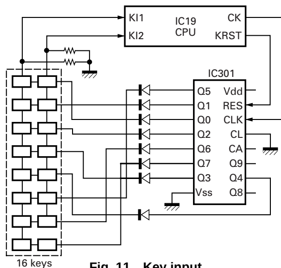
Fig. 11 Key input
