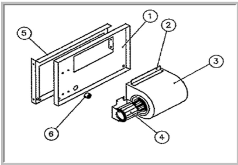
HL Fan Deck Assembly
