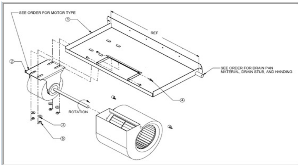
VL Fan Deck Assembly
