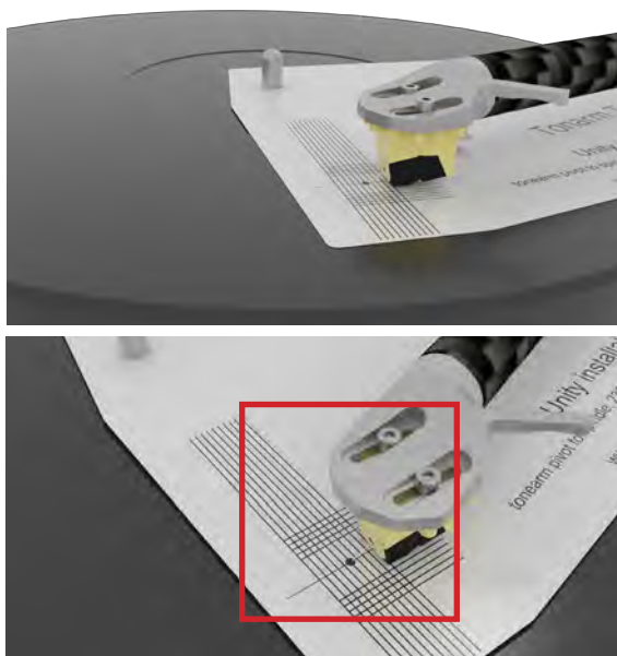
Abb. 19: Korrekte Ausrichtung des Tonabnehmers
