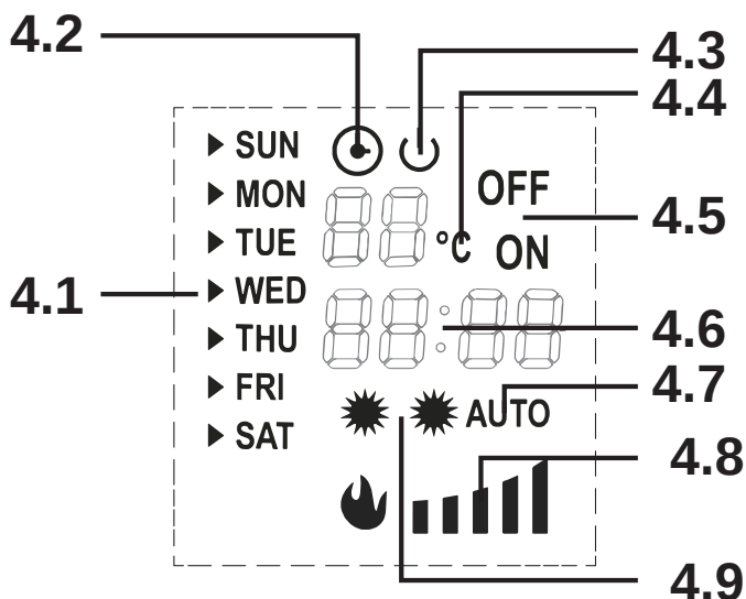
Écran LCD
