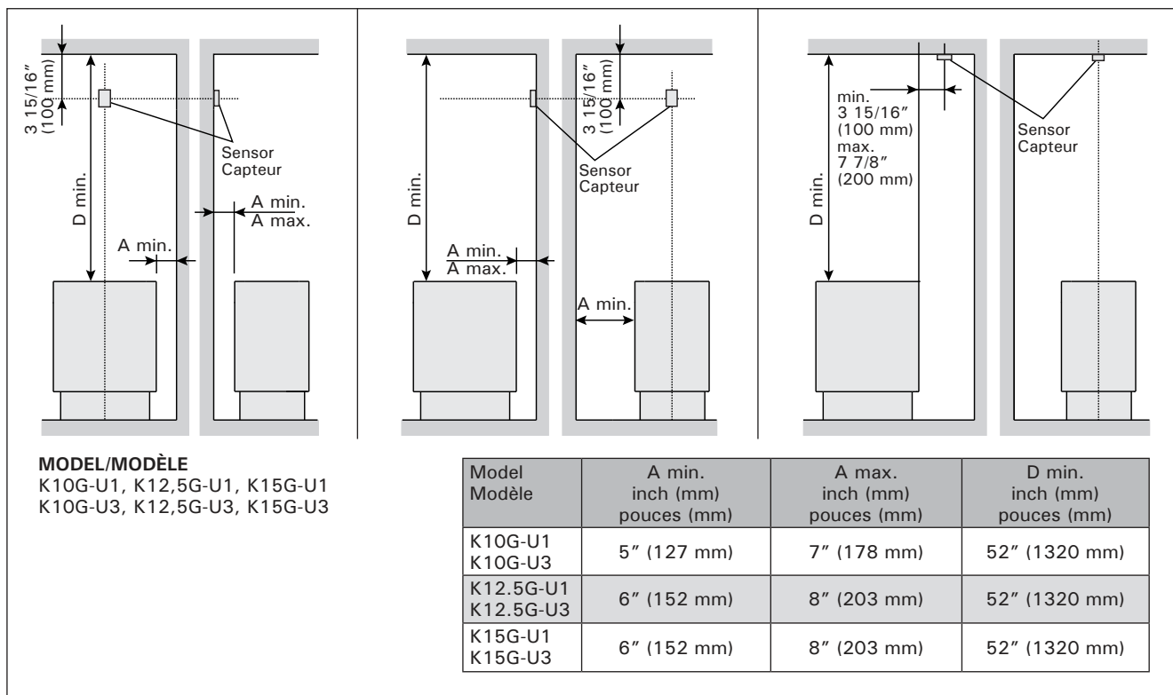
Figure 7. The place of the temperature sensor of the control unit in connection with floor-mounted heaters Figure 7. Emplacement des capteurs de température par rapport aux poêles en installation au sol
