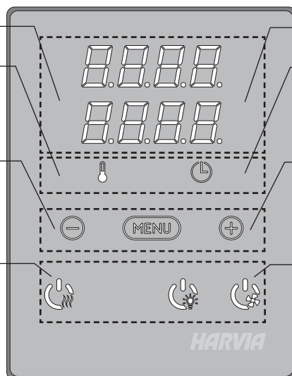
Figure 2. Le tableau de commande
