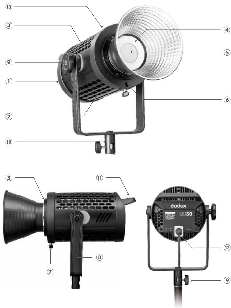
1.灯体 2.散热孔 3.保荣卡口 4.灯头保护罩 5.LED灯 6.伞孔 7.伞固定旋钮 8.U型支架 9.支架旋钮 10.支架套筒 11.把手 12.电源输入接口 13.卡口固定旋钮
