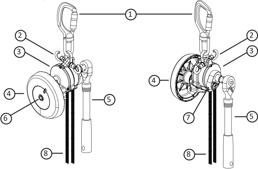
Figura 1: acerca del Dispositivo de Rescate y Descenso FallTech® UniDrive
