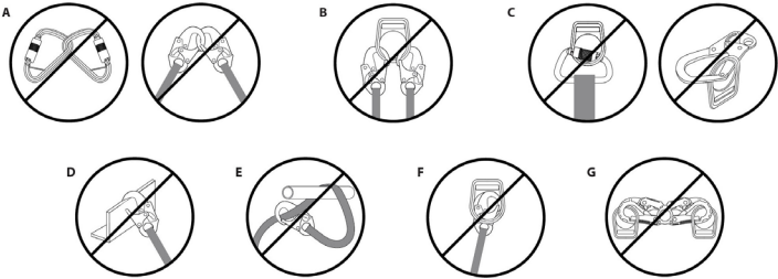
Figura 3 - Conexiones no compatibles
