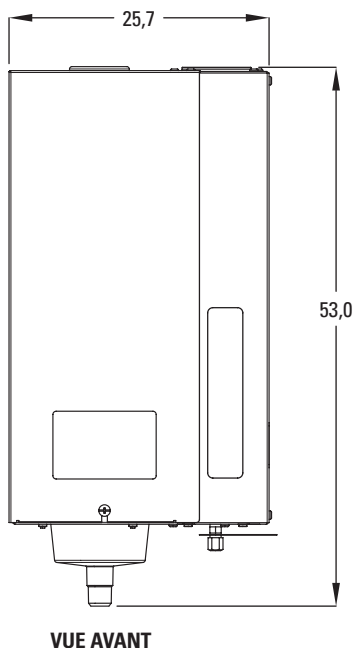
VUE AVANT
