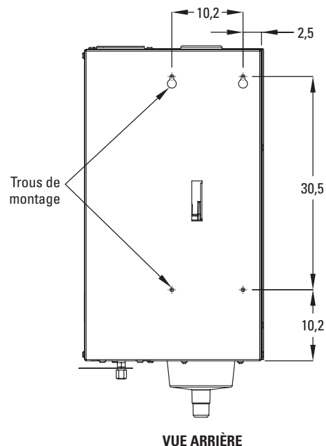
VUE ARRIÈRE
