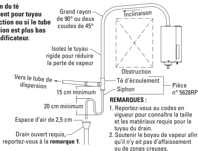
FIGURE 4 – Tube de dispersion monté sous l'humidificateur
