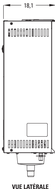
VUE LATÉRALE
