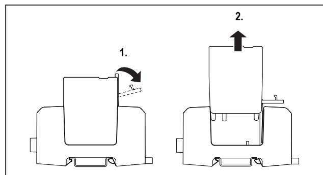
Bild 8.2 Überspannungsableiter entfernen
