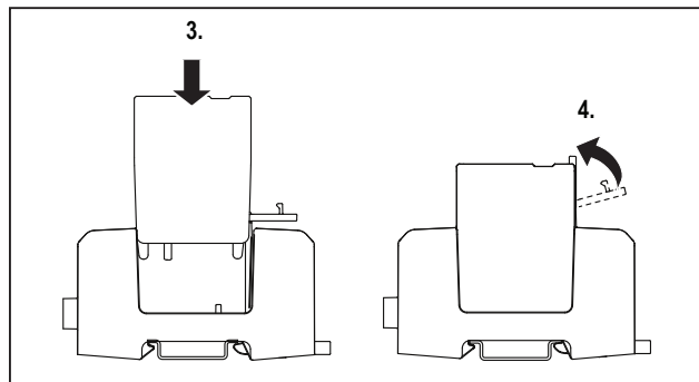
Bild 8.3 Überspannungsableiter einsetzen
