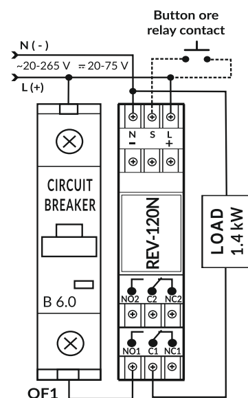
QF1 – Circuit breaker max 6 A
