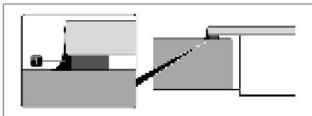
Fig. 11.26 Sellante de silicona para montaje superpuesto
