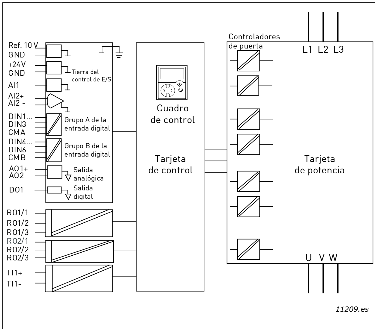
Figura 50. Barreras de aislamiento galvánico
