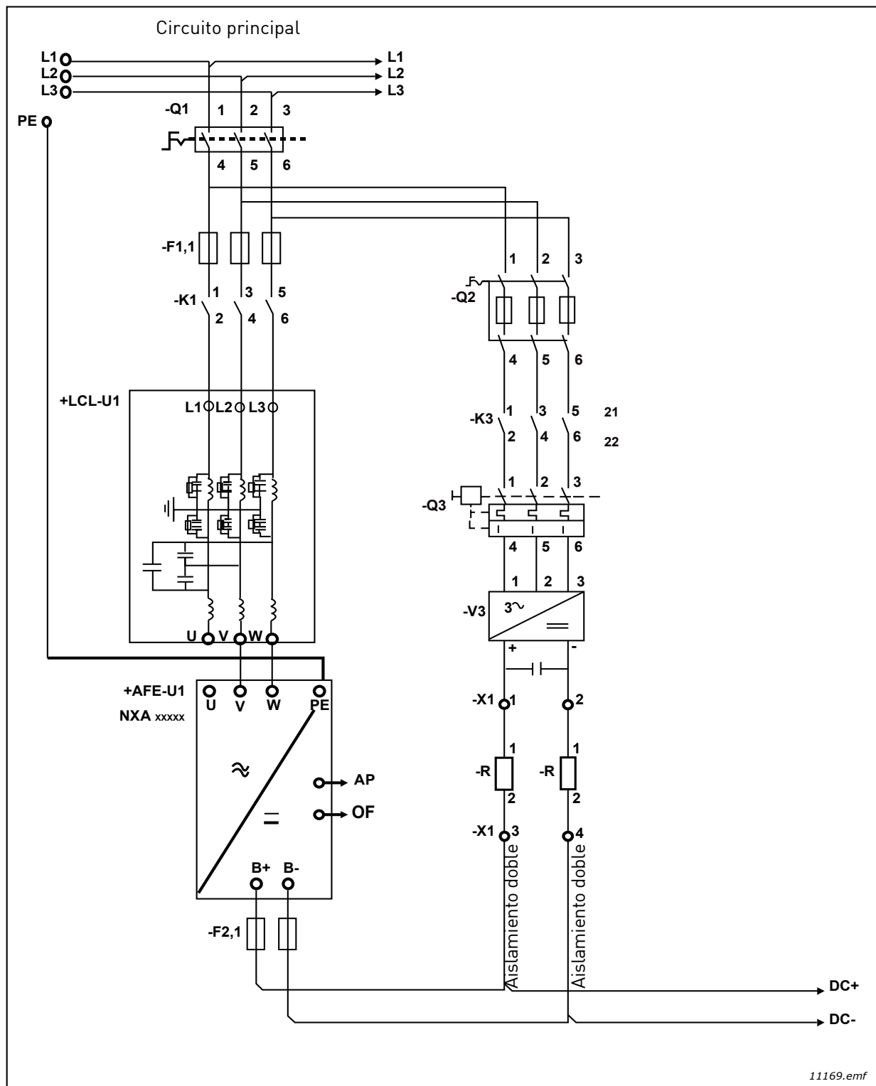
Figura 8. Conexiones para una sola unidad Vacon Active Front End
