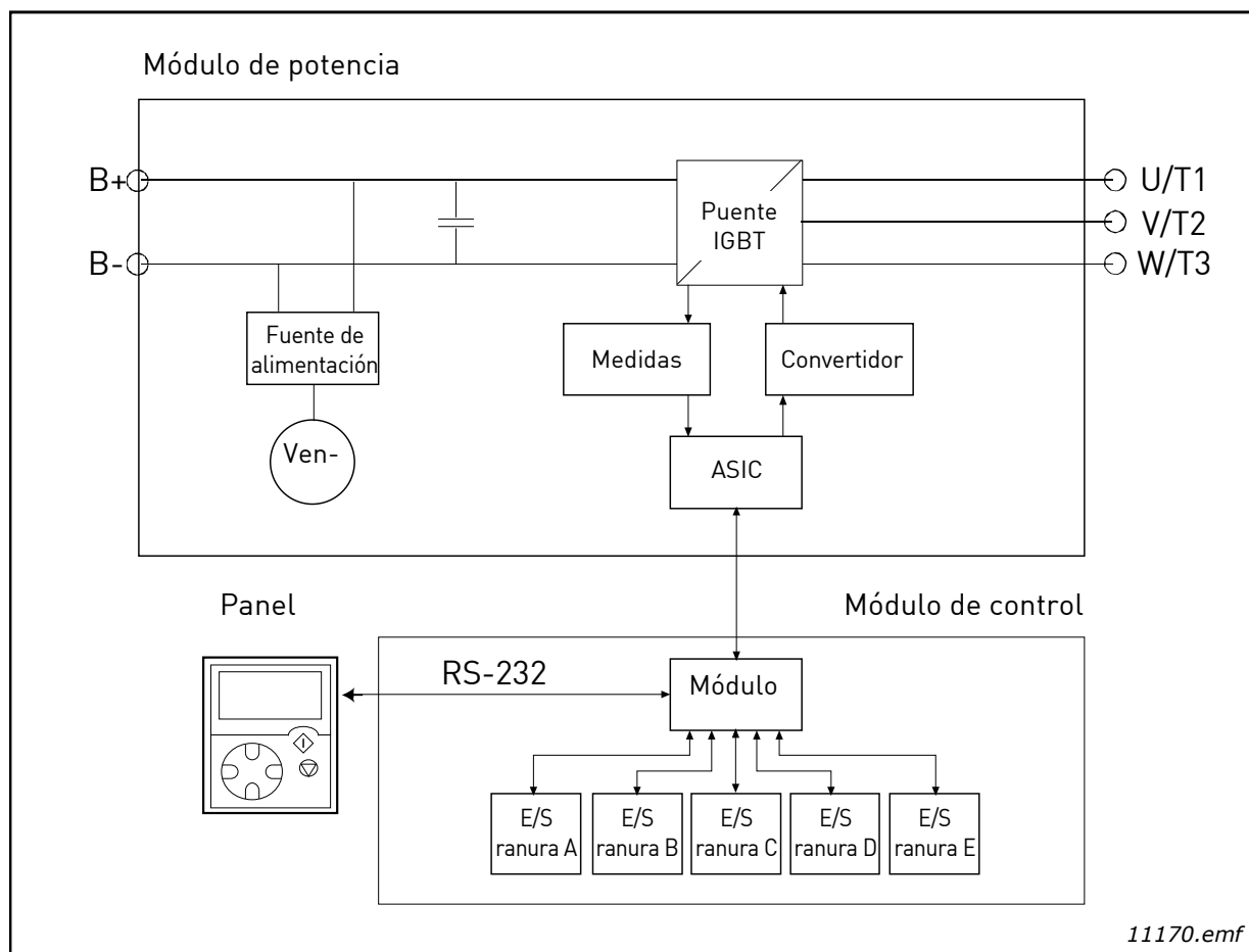
Figura 9. Diagrama de bloque de NXA
