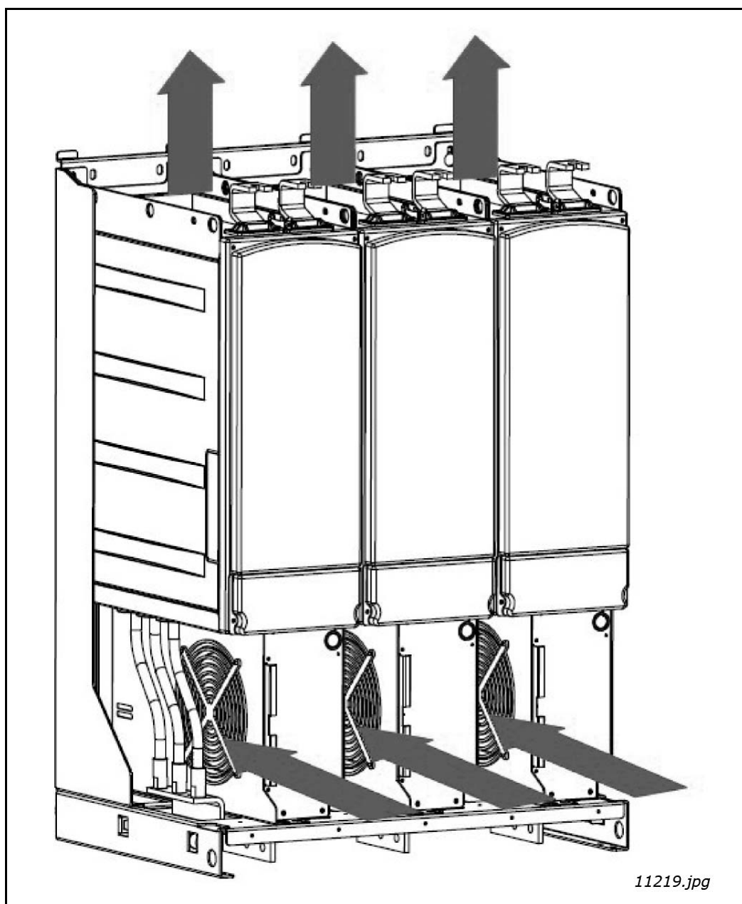
Figura 34. Flujo de aire de refrigeración para la unidad FI13
