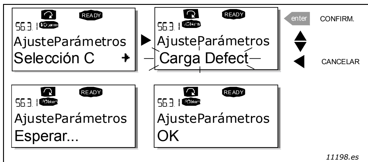
Figura 59. Almacenar y cargar conjuntos de parámetros
