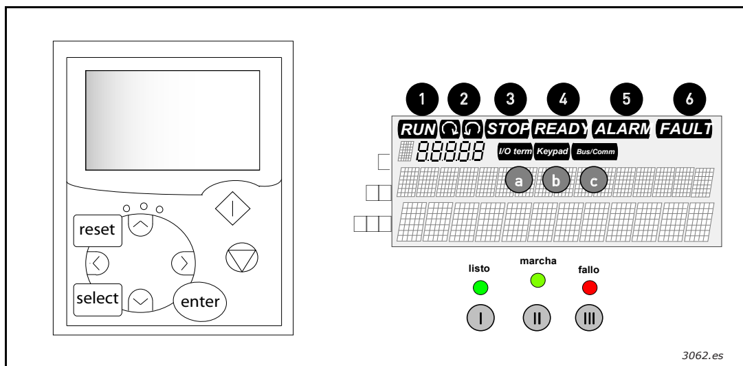
Figura 51. Panel de control del inversor Vacon e indicaciones sobre el estado de la unidad
