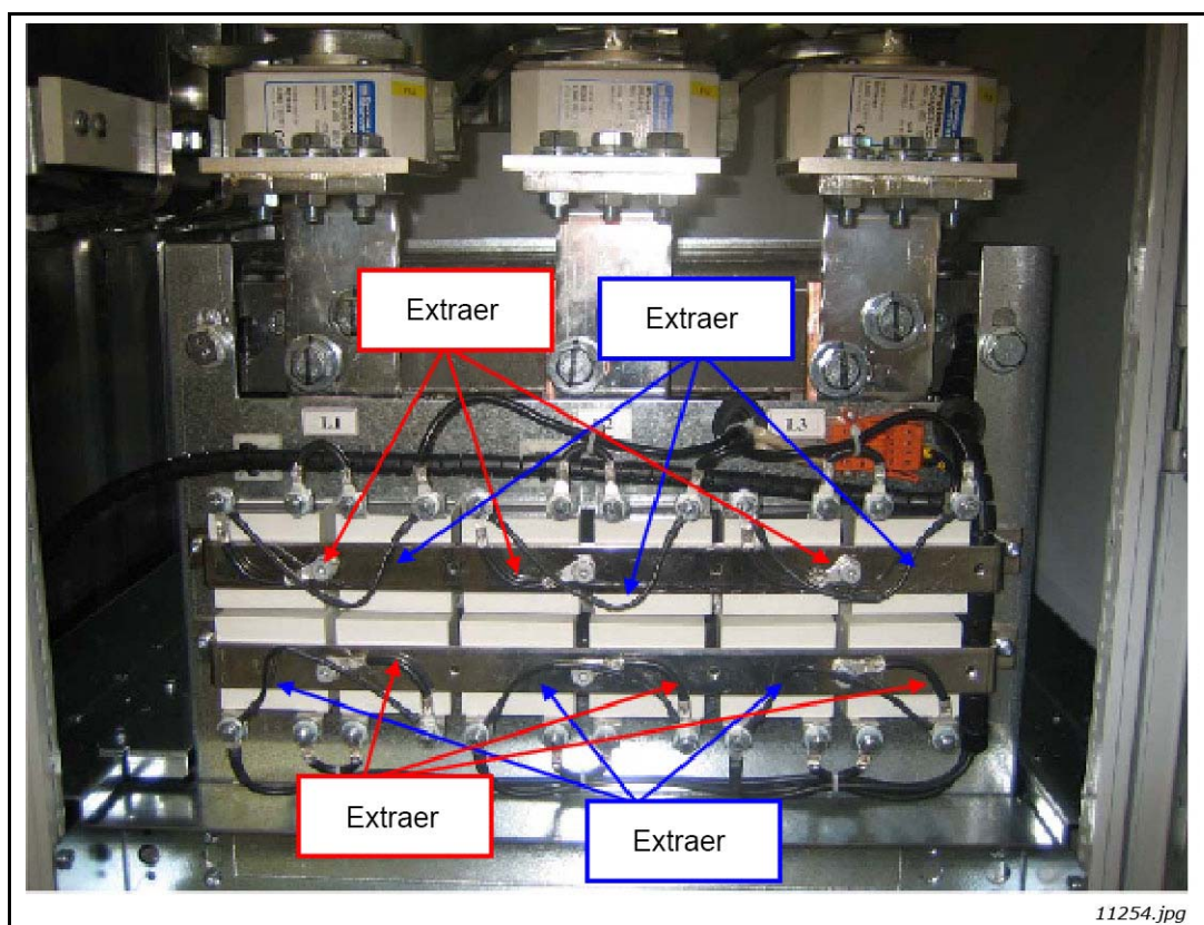
Figura 19. Condensadores de HF en el filtro LCL de FI13
