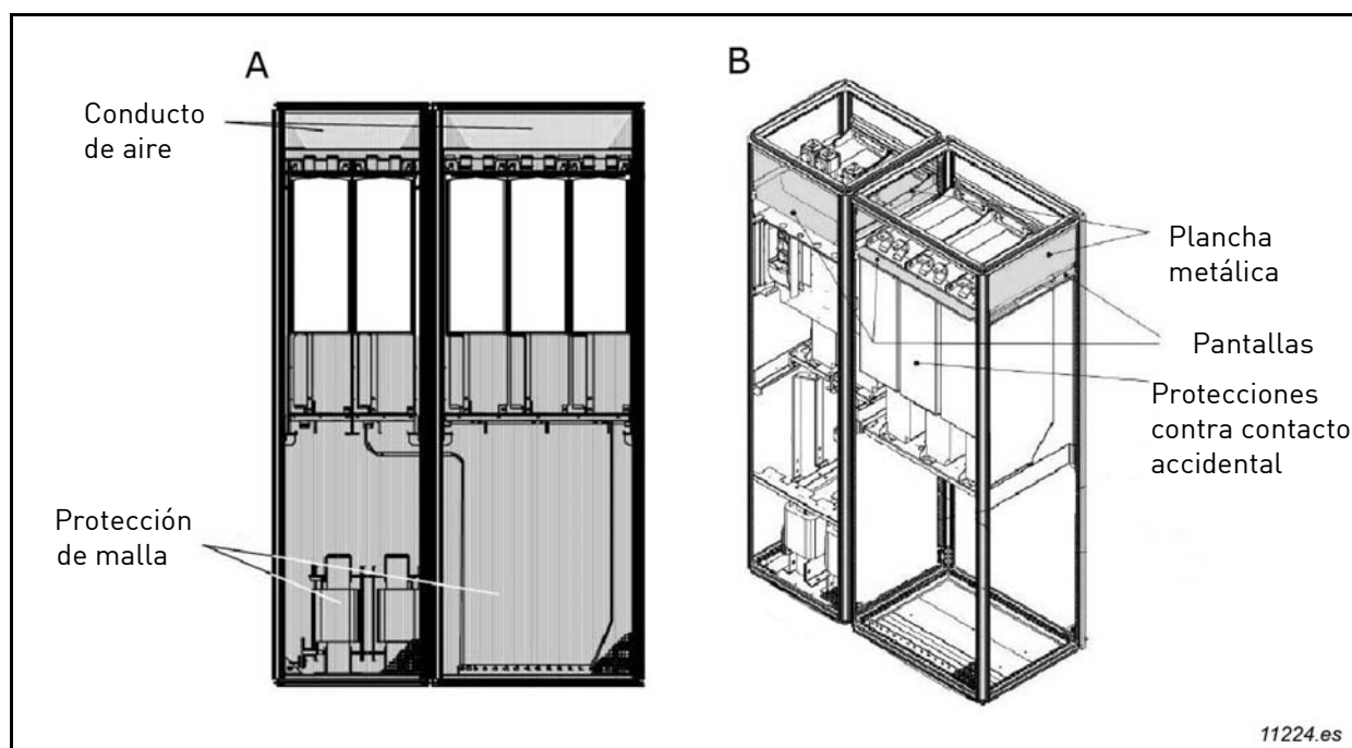
Figura 39. Guía para el flujo de aire de refrigeración del armario
