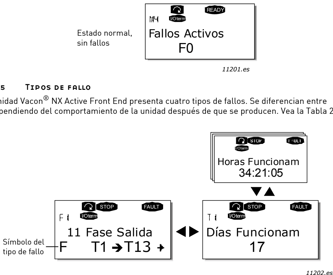
Figura 56. Fallo en pantalla
