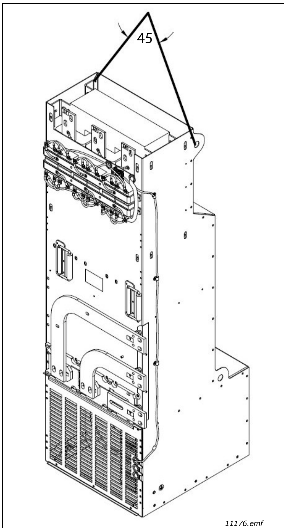
Figura 6. Puntos de elevación de los filtros LCL FI13
