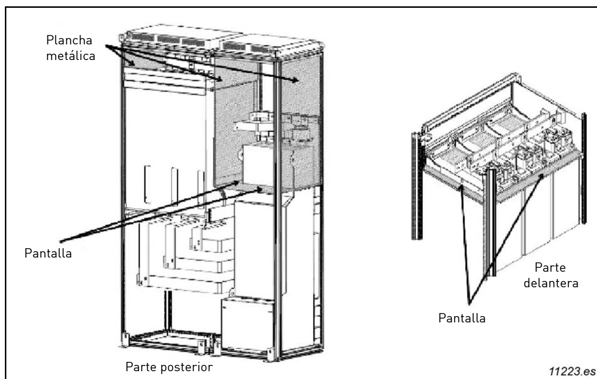
Figura 42. Guías de flujo de aire de refrigeración del armario para la unidad AFE FI13 y el filtro LCL
