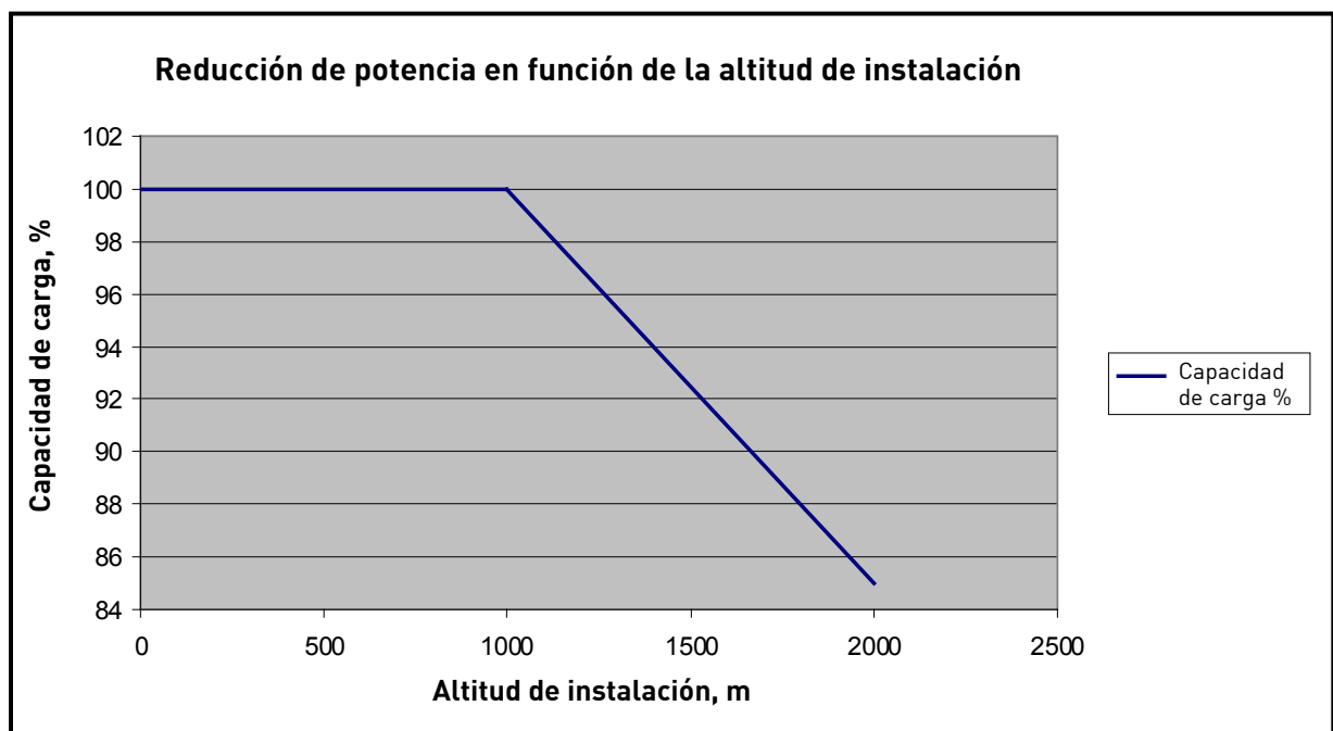
Figura 24. Reducción de potencia en función de la altitud de instalación, 525–690 V
