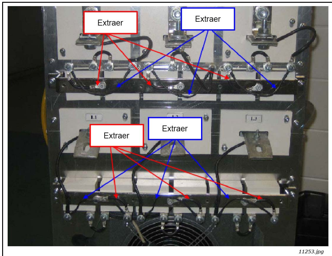
Figura 18. Condensadores de HF en el filtro LCL de FI9 y FI10
