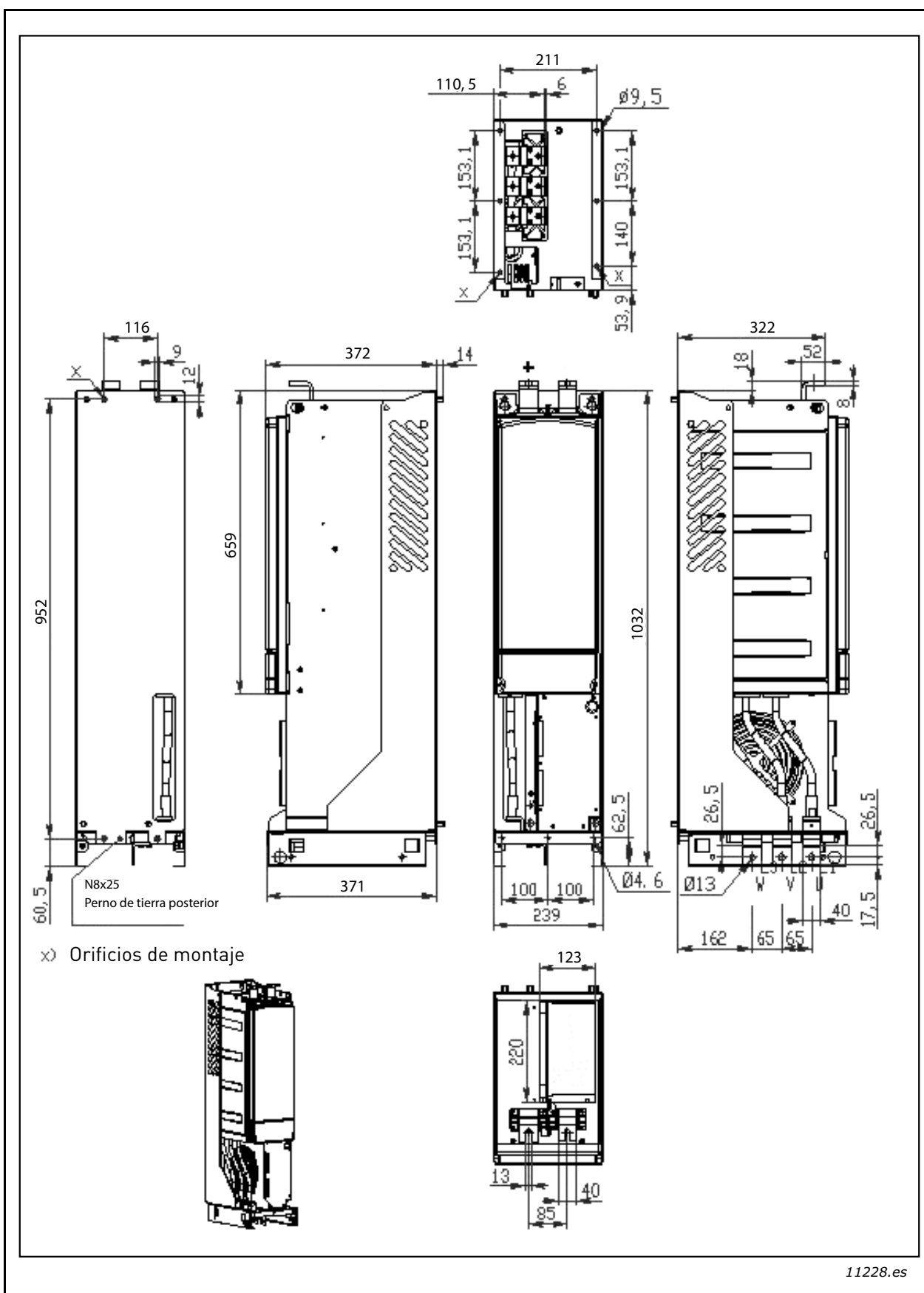
Figura 72. Dimensiones de la unidad FI9
