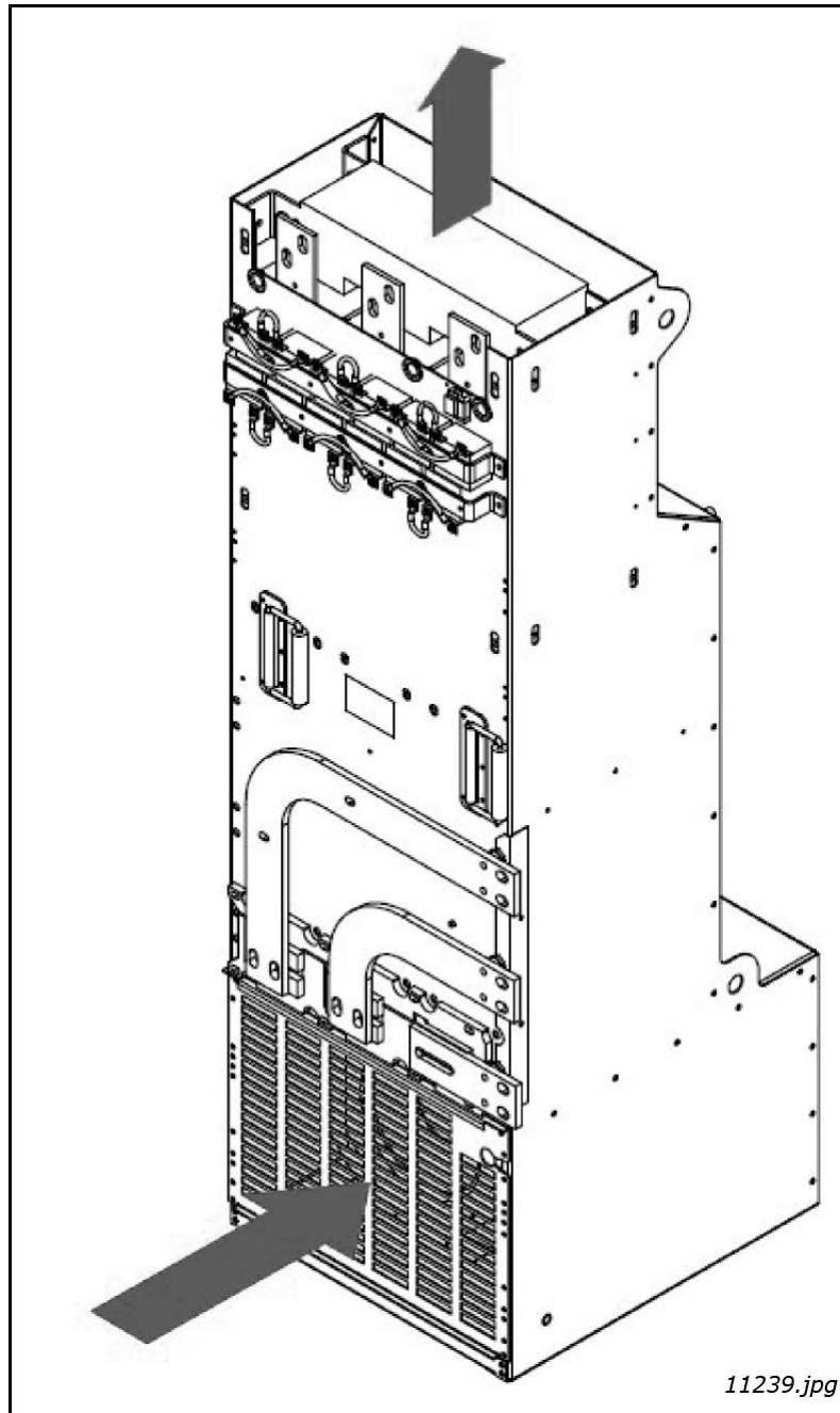
Figura 37. Guías de flujo de aire de refrigeración para el filtro LCL de la unidad FI13
