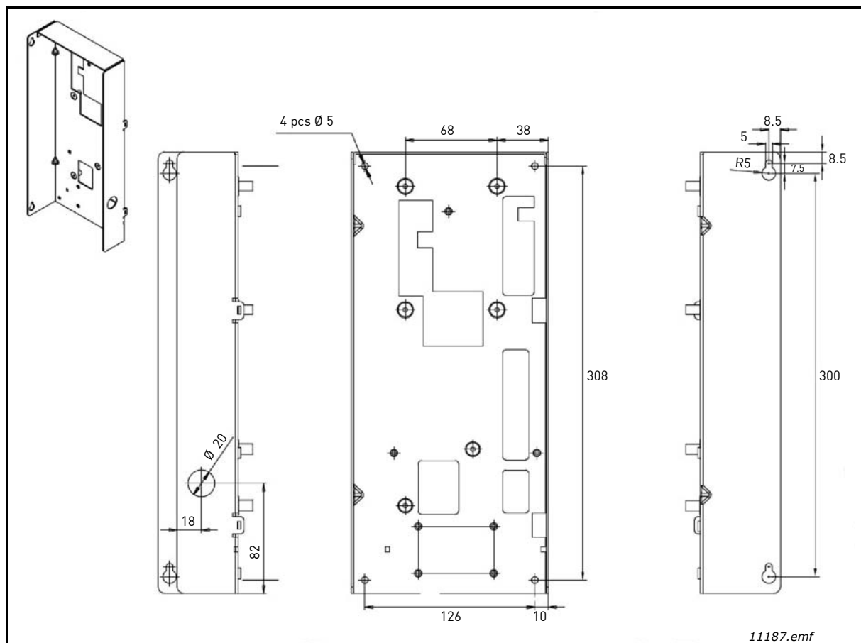
Figura 31. Puntos de montaje de la caja de control
