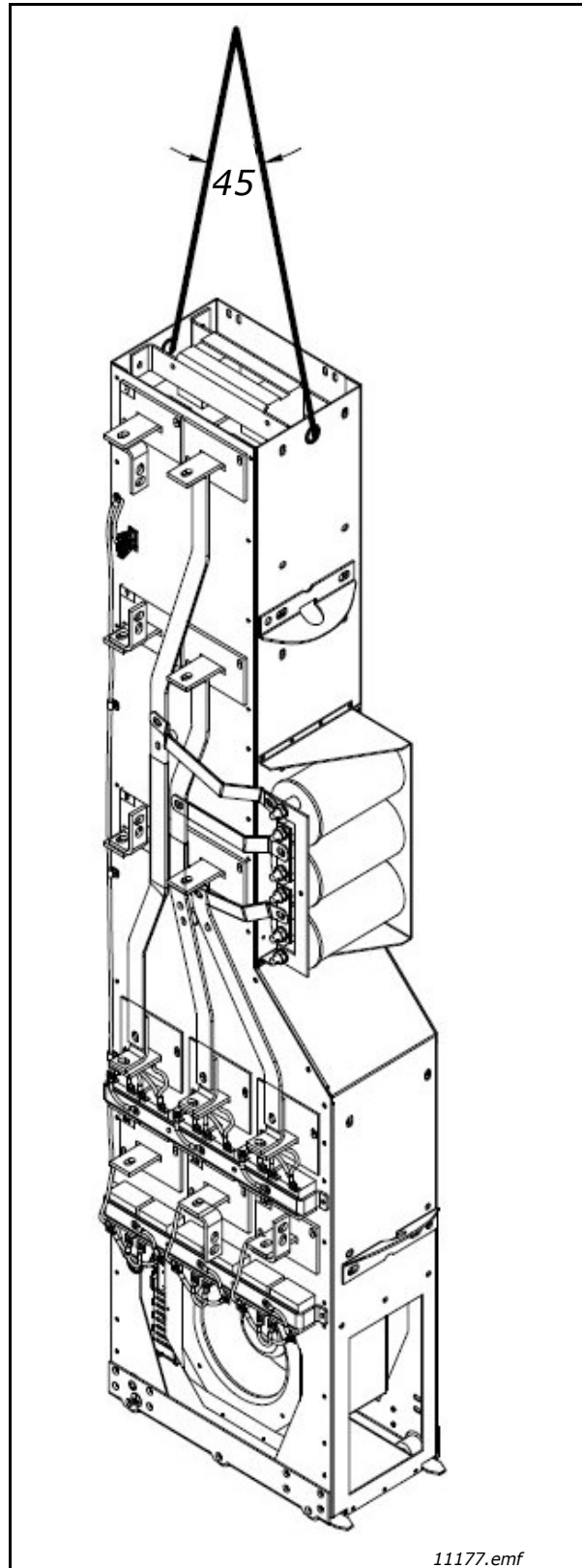
Figura 5. Puntos de elevación de los filtros LCL FI9 y FI10
