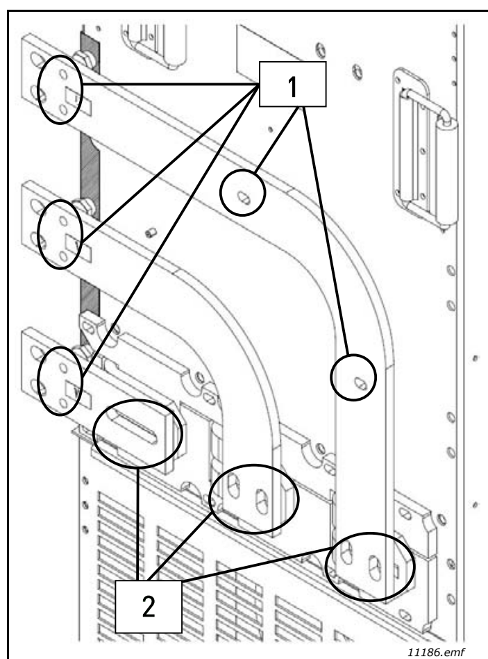
Figura 29. Conexión hacia la izquierda
