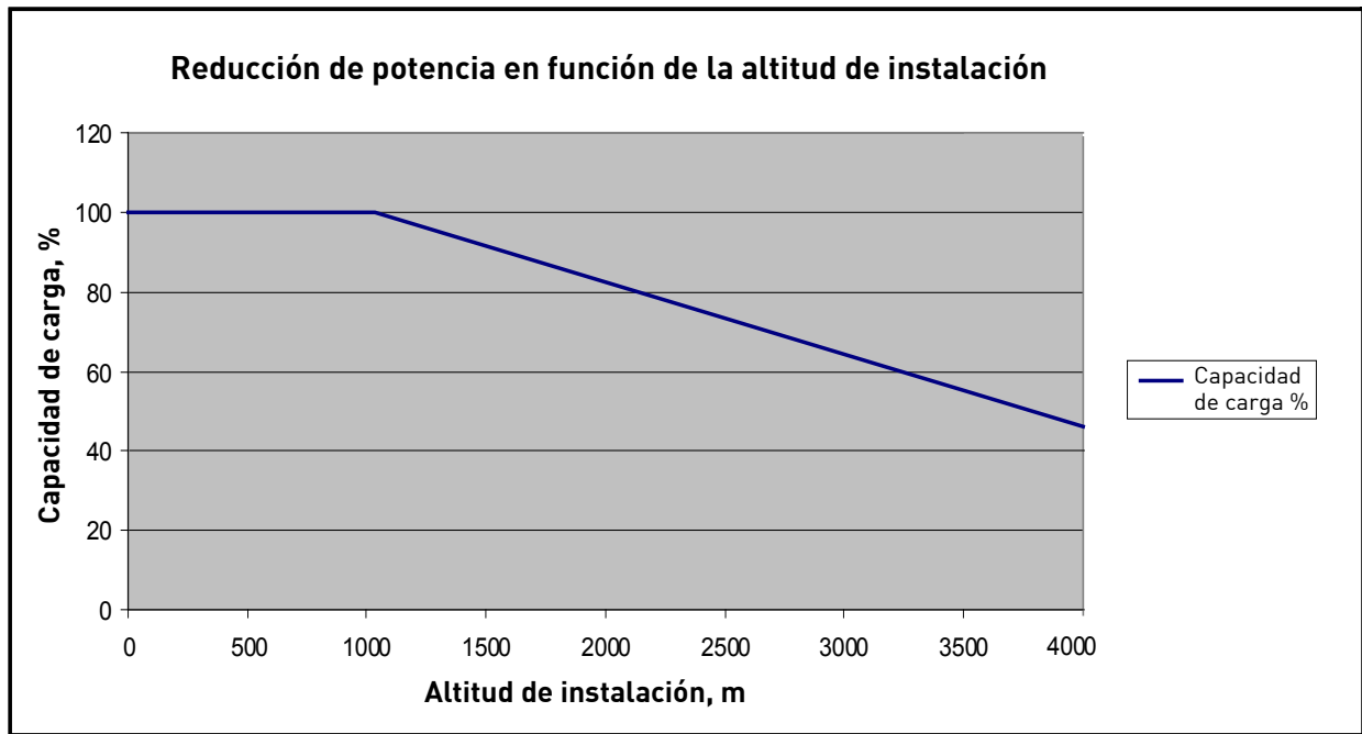
Figura 23. Reducción de potencia en función de la altitud de instalación, 380–500 V
