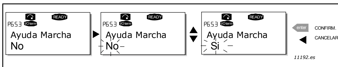
Figura 64. Activación del asistente de arranque
