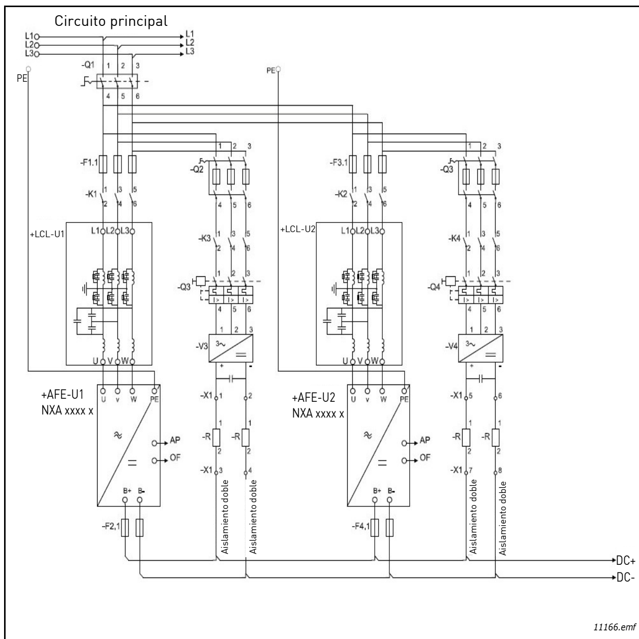
Figura 21. Conexión de unidades Active Front End en paralelo con sus propios circuitos de precarga
