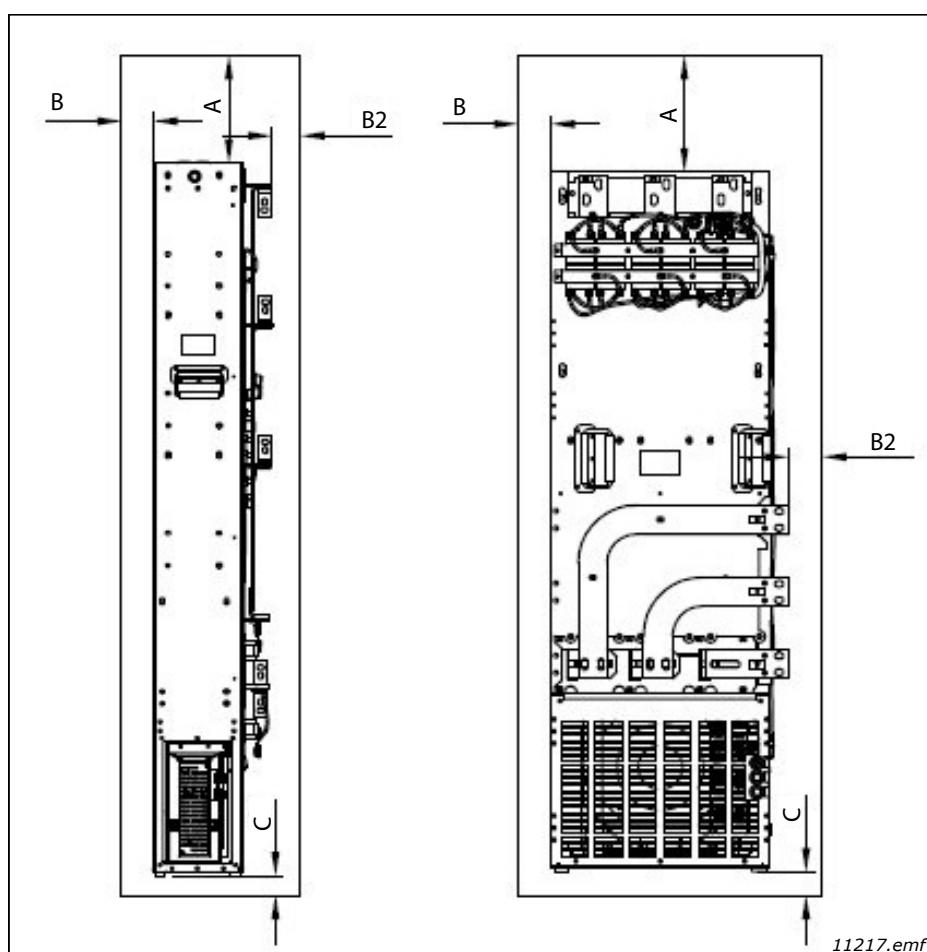
Figura 35. Espacio para la instalación
