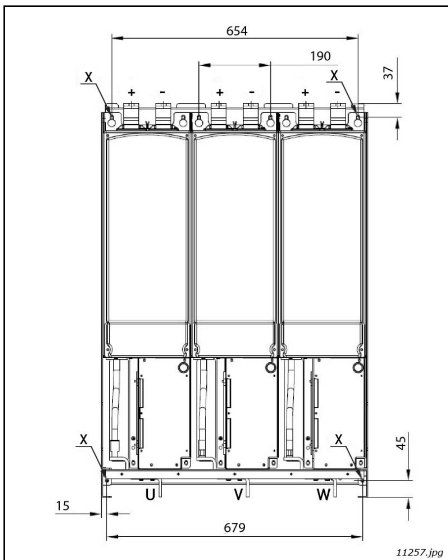
Figura 27. Puntos de montaje de la unidad AFE FI13
