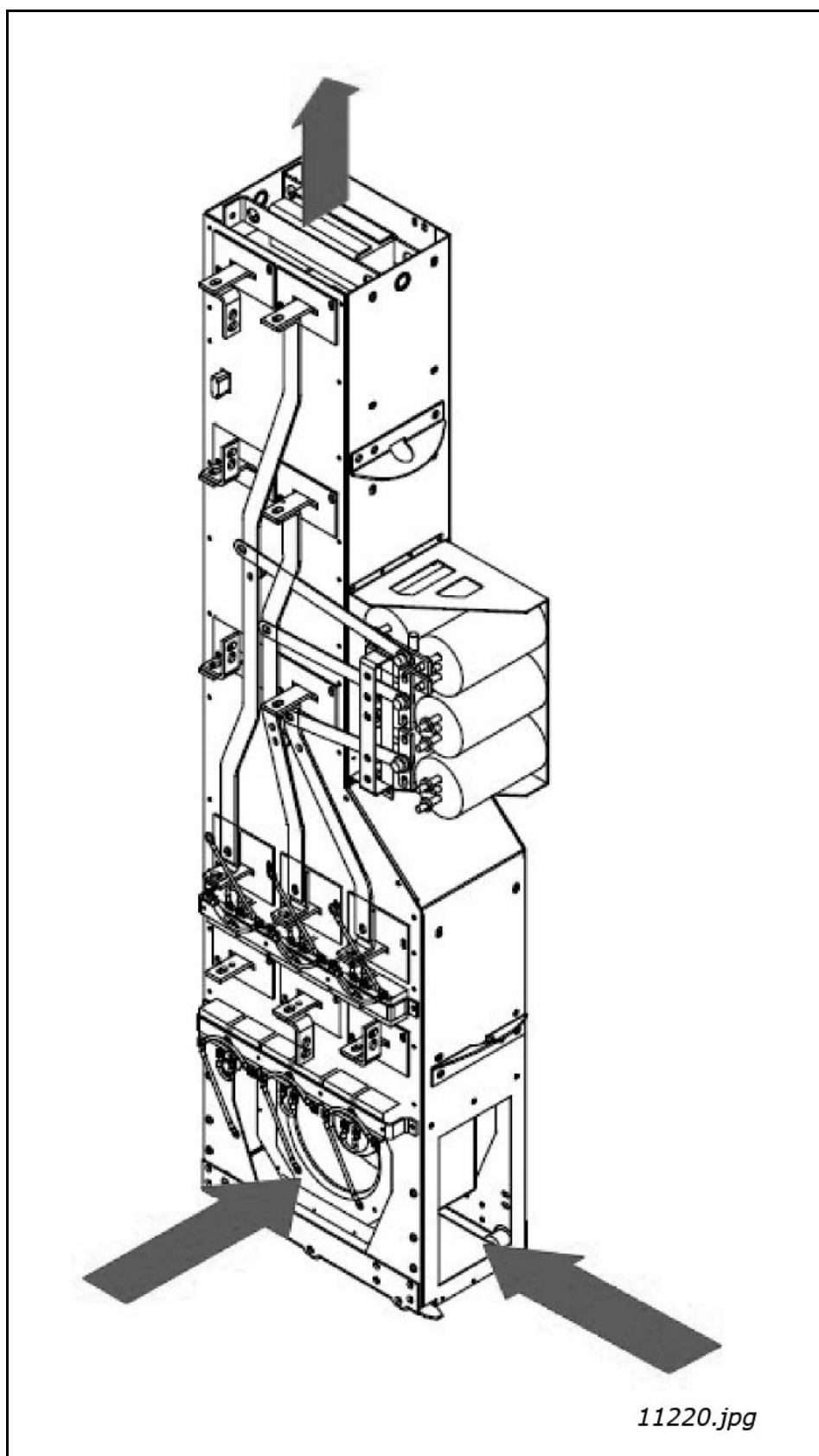
Figura 36. Flujo de aire de refrigeración para los filtros LCL de las unidades FI9 y FI10
