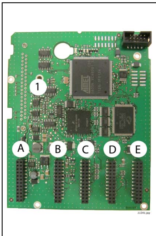
Figura 48. Tarjeta de control
