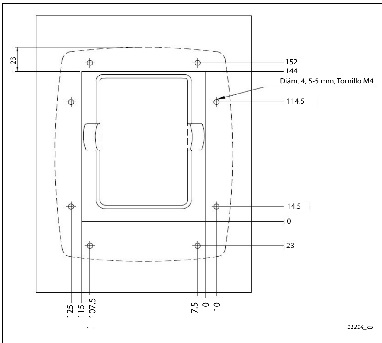
Figura 81. Dimensiones del kit de montaje de la puerta
