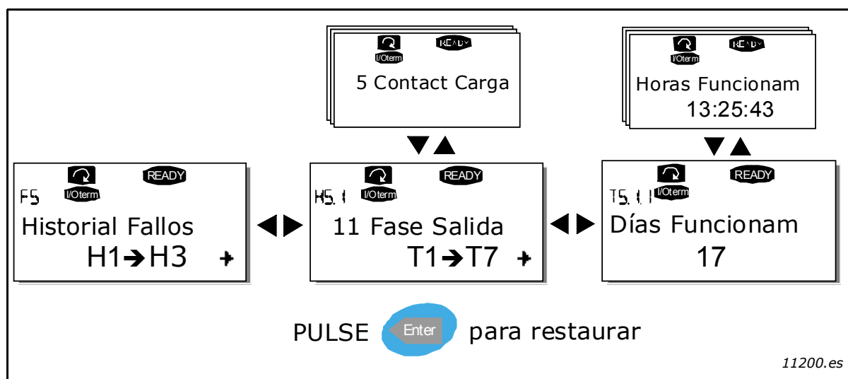
Figura 57. Menú del historial de fallos
