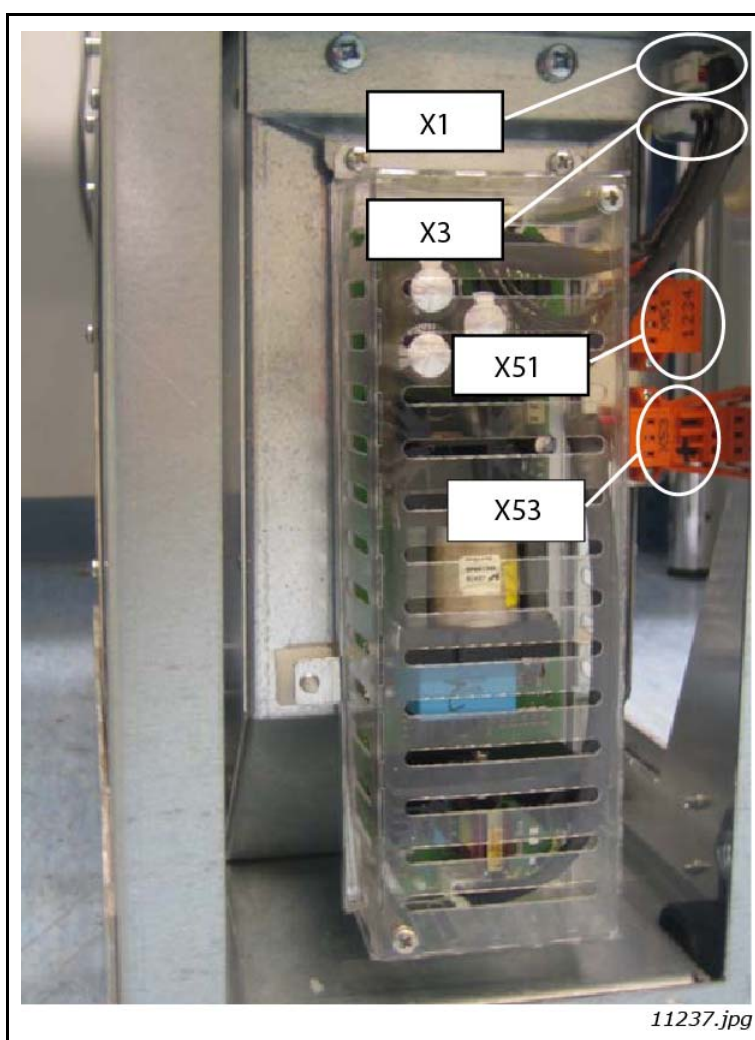
Figura 43. Alimentación de CC/CC integrada en el filtro LCL FI9 y FI10
