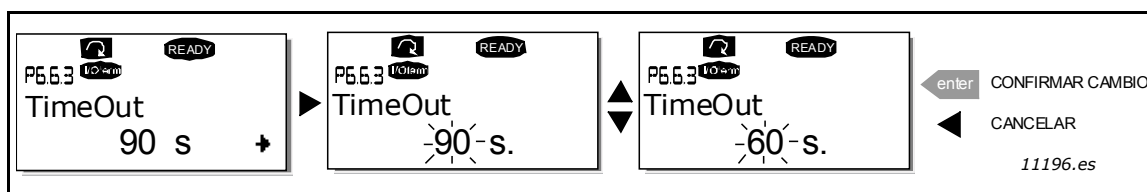
Figura 68. Establecer la configuración tiempo de espera
