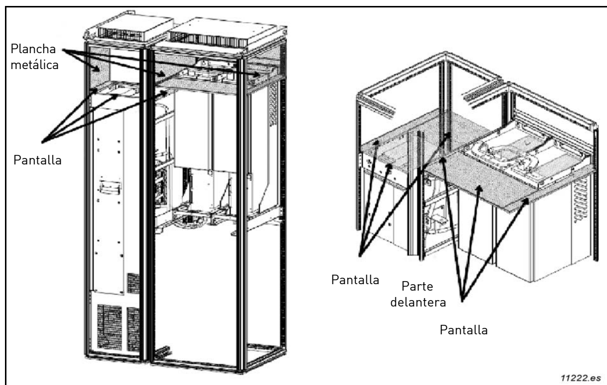
Figura 41. Guías de flujo de aire de refrigeración del armario para las unidades AFE FI9 y FI10 y el filtro LCL
