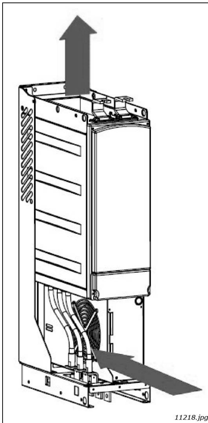
Figura 33. Flujo de aire de refrigeración para las unidades FI9 y FI10
