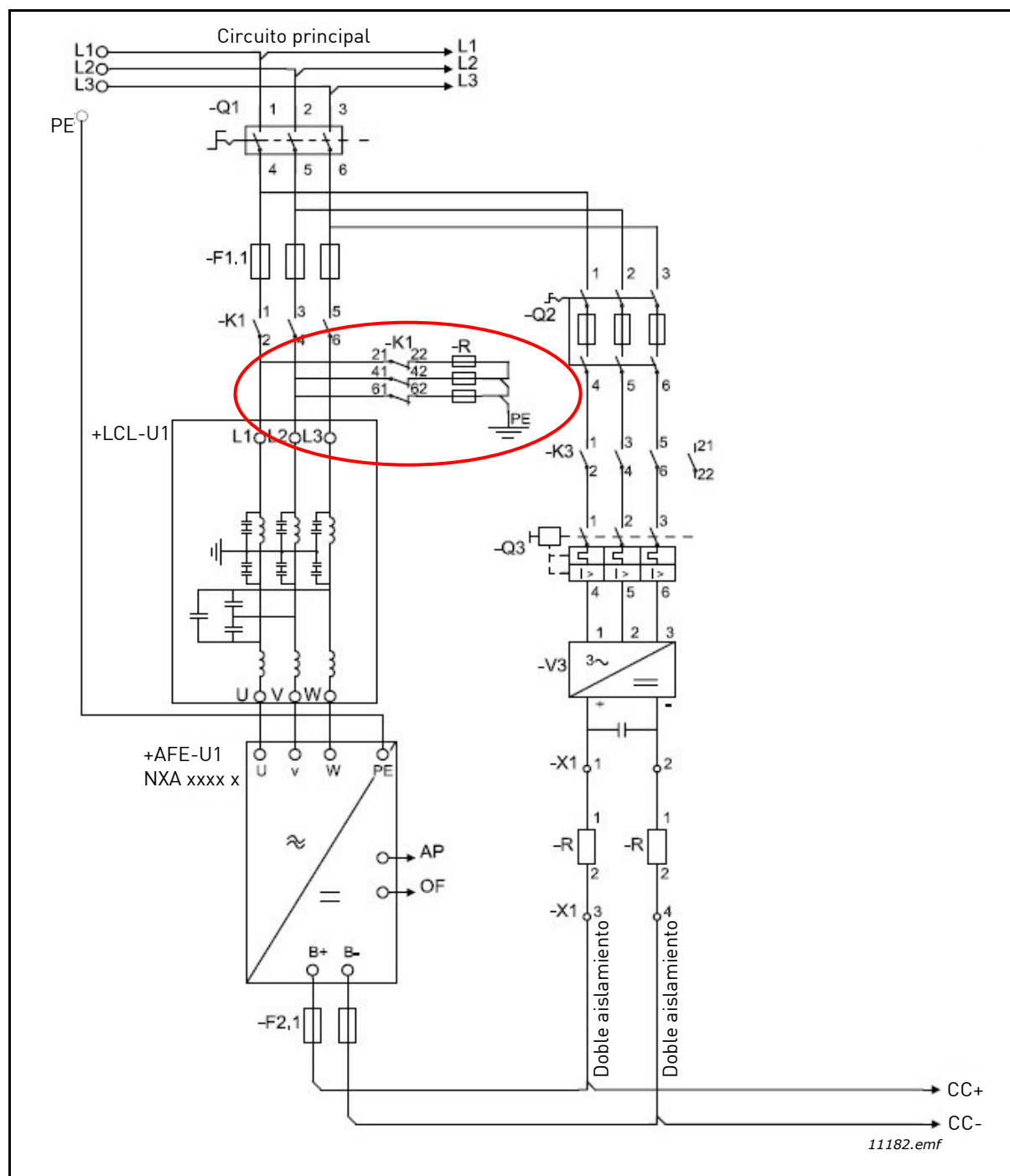
Figura 17. Diagrama de cableado del circuito de descarga alternativo
