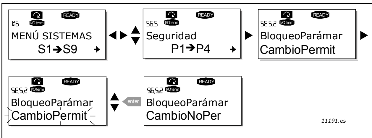
Figura 63. Bloqueo de parámetros
