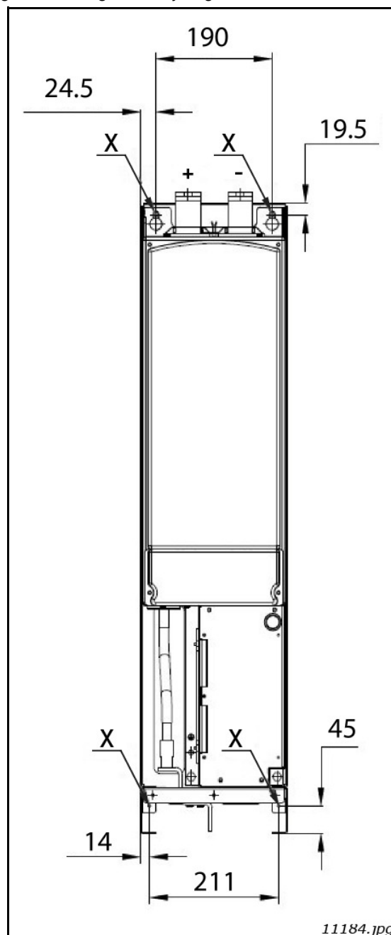
Figura 25. Puntos de montaje de la unidad AFE FI9
