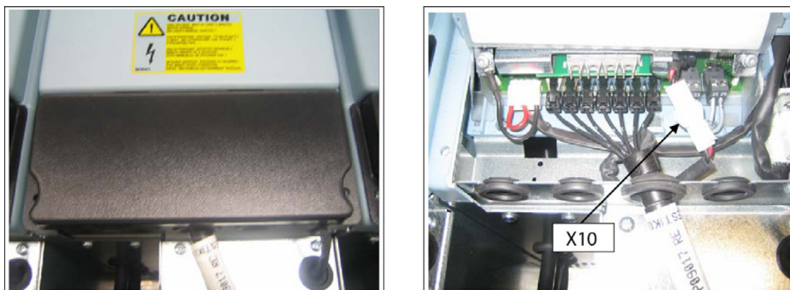
Figura 15. Terminales de cable óptico de la unidad (ejemplo FI13)
