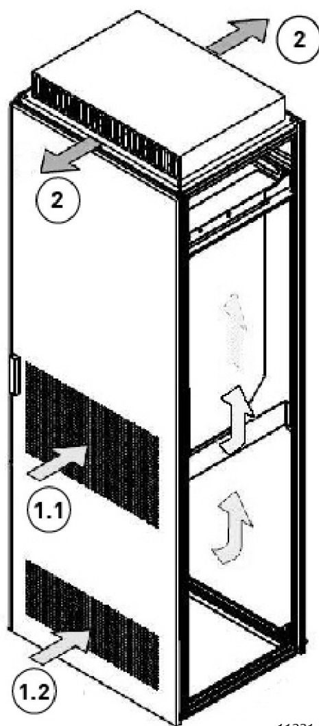
Figura 38. Aberturas del armario para refrigeración
