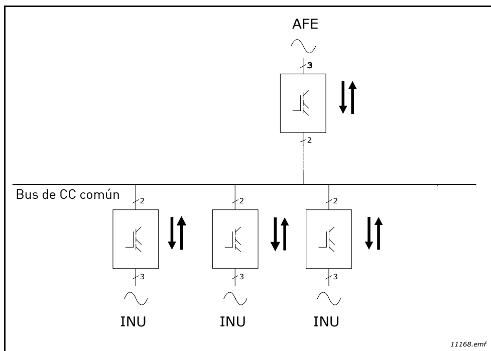
Figura 7. Configuración típica de una unidad Active Front End
