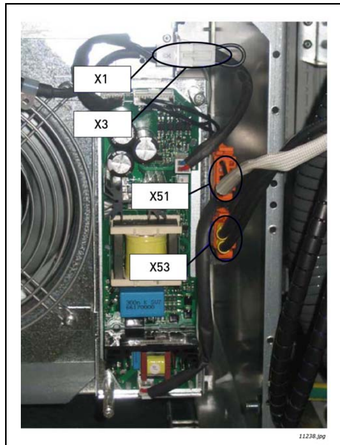
Figura 44. Alimentación de CC/CC integrada en el filtro LCL FI13
