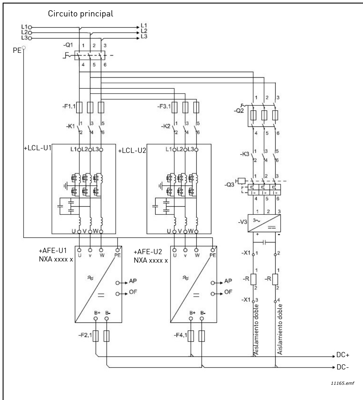
Figura 20. Conexión de unidades Active Front End en paralelo con un circuito de precarga común
