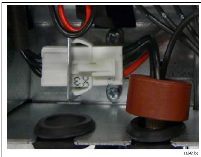
Figura 46. Terminal X3 (fase U en FI13) en la unidad
