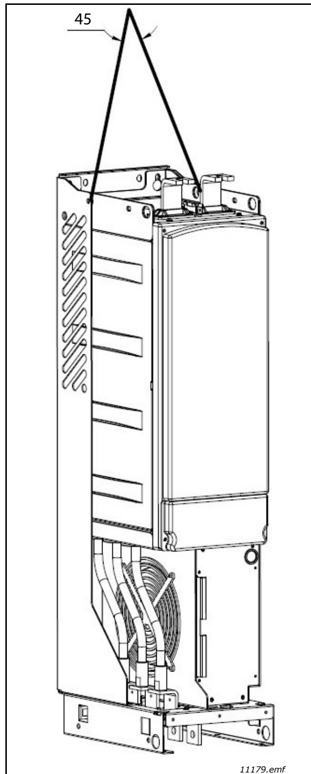
Figura 3. Puntos de elevación de los módulos FI9 y FI10
