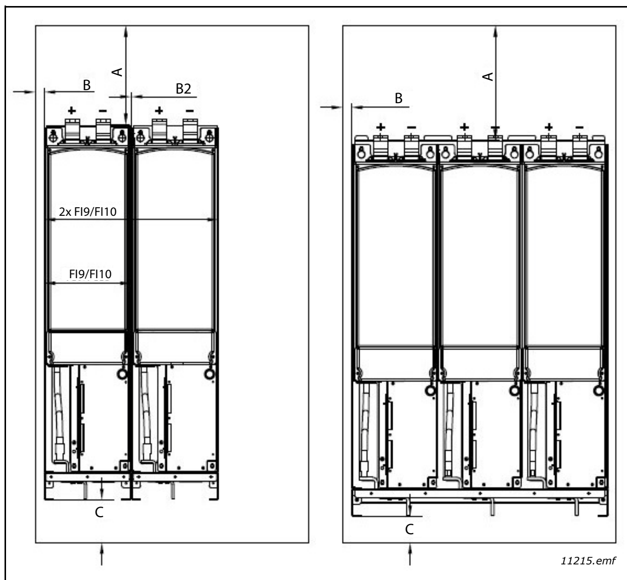
Figura 32. Espacio de instalación para las unidades FI9, FI10 y FI13
