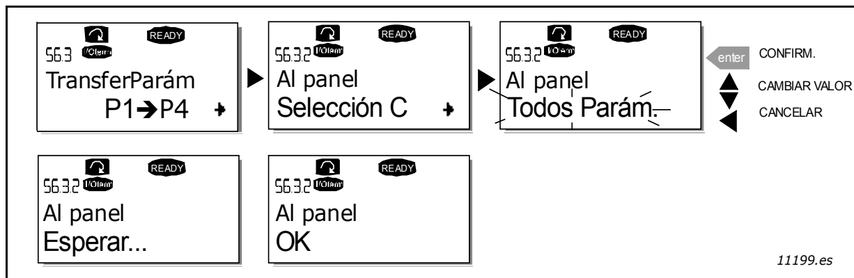
Figura 60. Copia de parámetros en el panel
