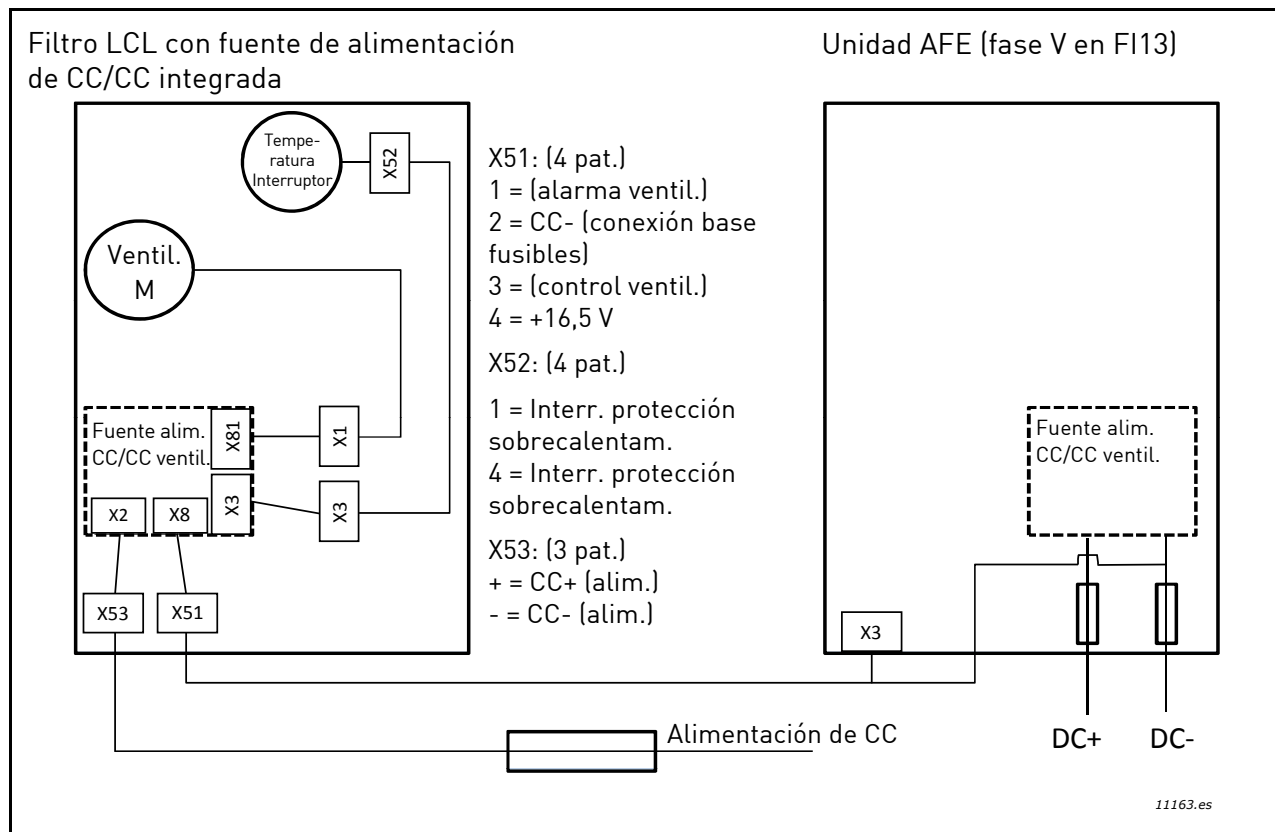
Figura 45. Diagrama de cableado de la alimentación de CC/CC integrada
