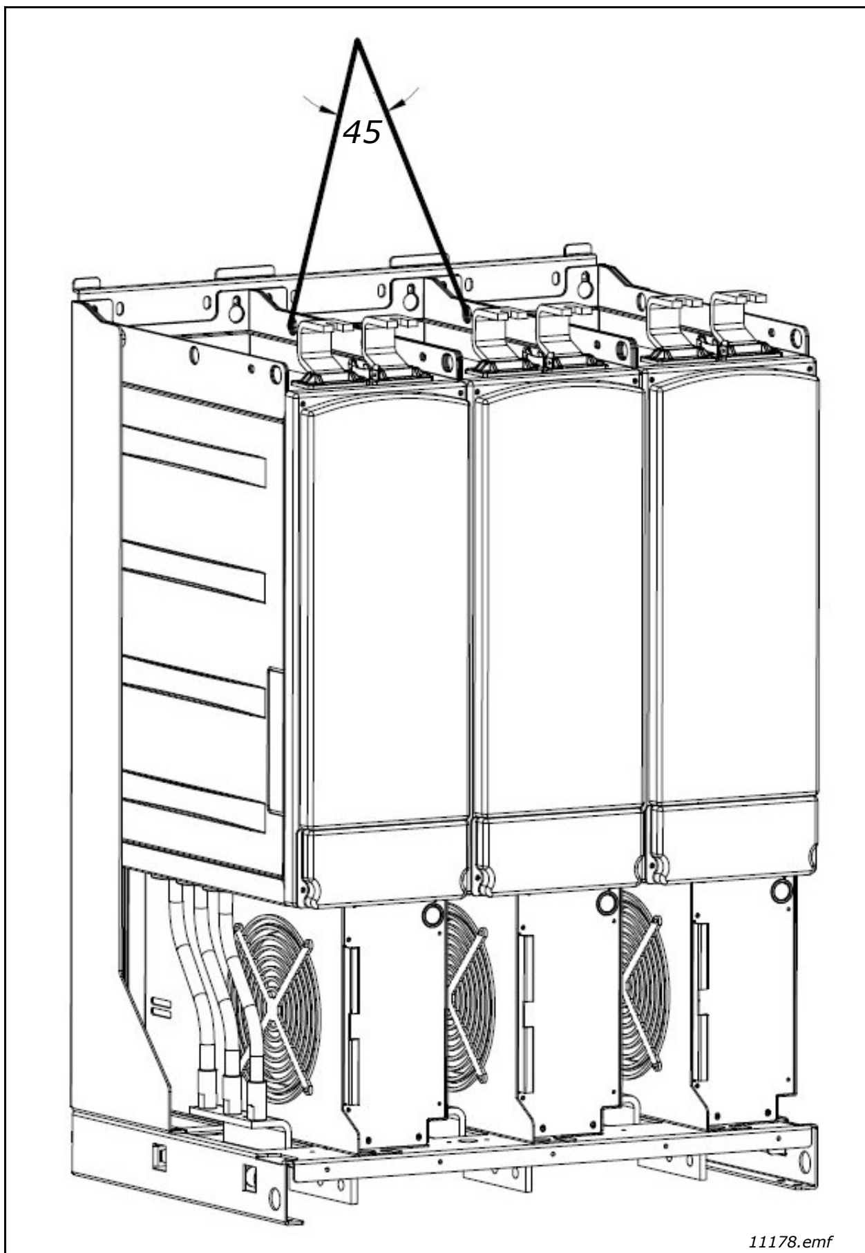
Figura 4. Puntos de elevación de los módulos FI13
