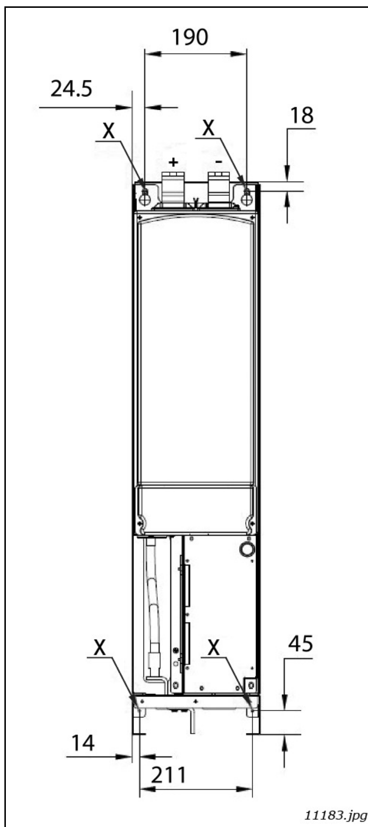
Figura 26. Puntos de montaje de la unidad AFE FI10
