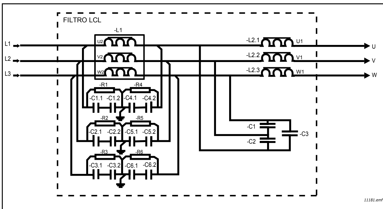
Figura 16. Diagrama de cableado del filtro LCL de Vacon
