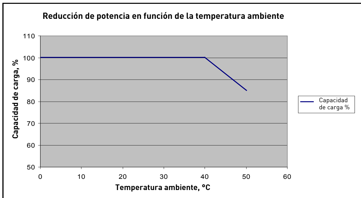
Figura 22. Reducción de potencia en función de la temperatura ambiente
