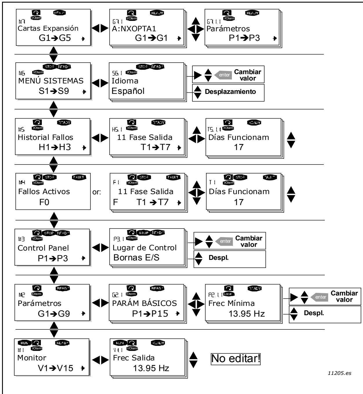
Figura 53. Cuadro de navegación del panel
