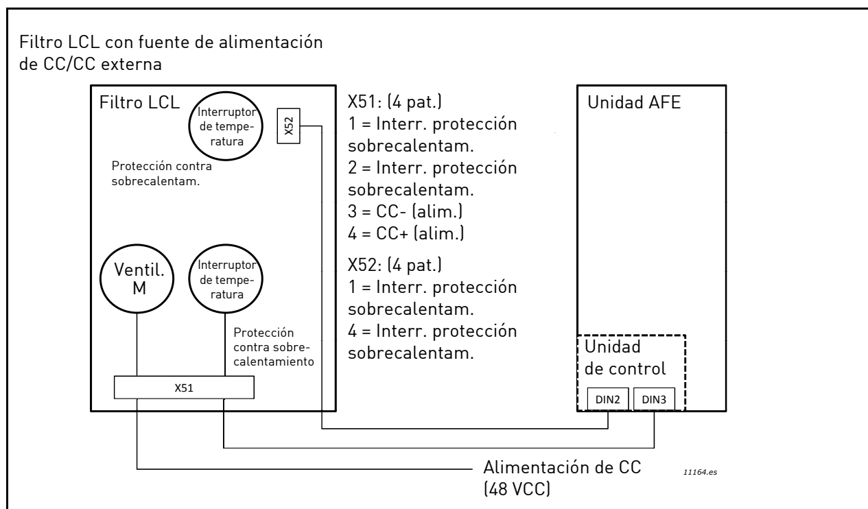
Figura 47. Diagrama de cableado de la alimentación de CC externa
