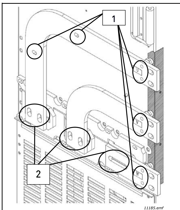
Figura 28. Conexión hacia la derecha
