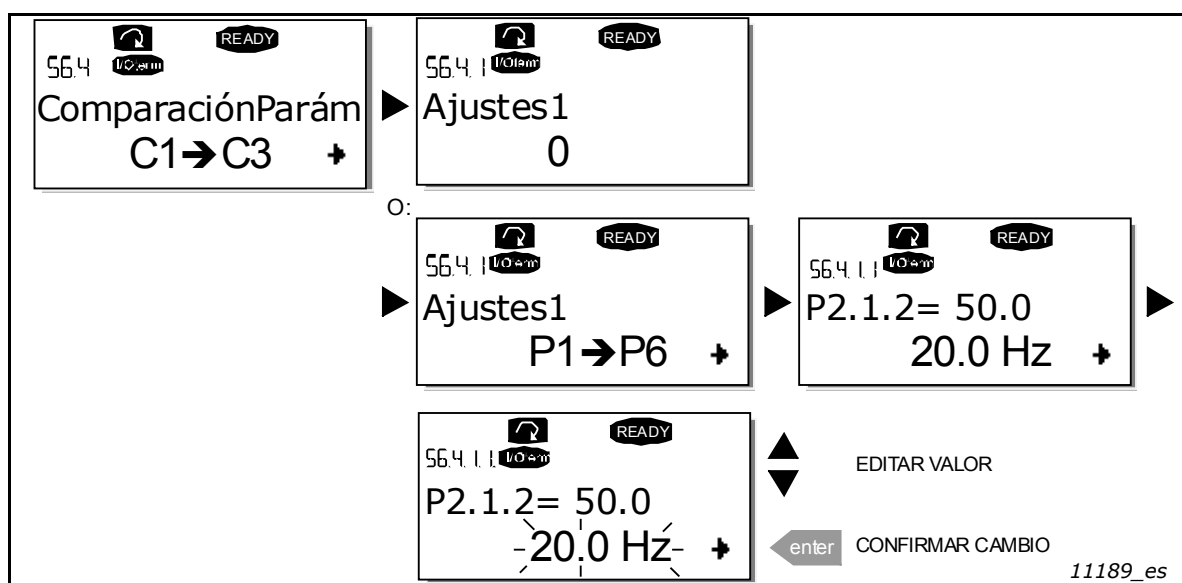
Figura 61. Comparación de parámetros
