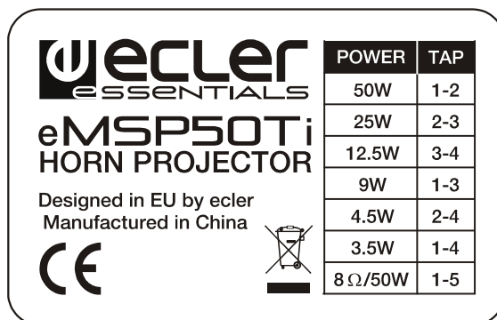
Abbildung 1: Anschlussdiagramm
