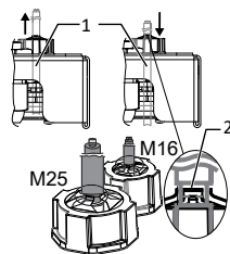
Imm. 14: Supporto di schermatura su pressacavi EMC
