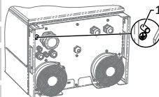
Rys. 12: Dodatkowy punkt uziemienia
