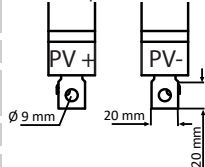
Sl. 10: Priklop na različico S
