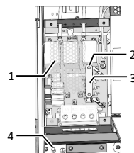
Fig. 3: 5-ledaranslutning
