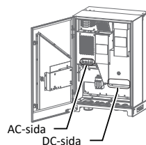
Fig. 7: Anslutningsklämmor:
