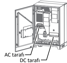
Şek. 7: Bağlantı klemensleri
