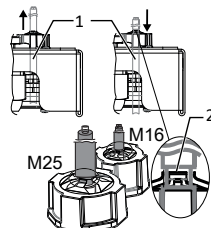
Sl. 14: Podloga oplaščenja na privitju EMV
