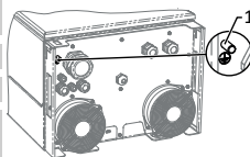
Sl. 12: Dodatna ozemljitvena točka
