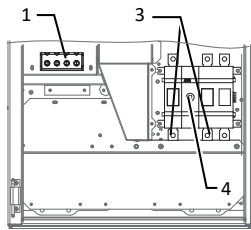
Fig. 4: Tilkoblingsklemmer - Basic-versjon
