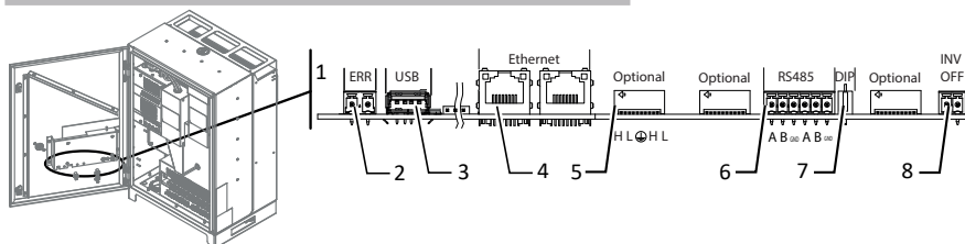
III. 13: Platine de communication : raccordement et affectation des interfaces
