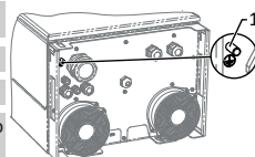
Fig. 12: Punto de toma a tierra adicional
