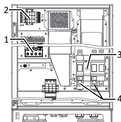
Fig. 5: Tilslutningsklemmer M-version
