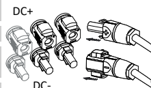
Fig. 11: Tilkobling på variant XL
