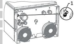
Kuva 12: Lisämaadoituspiste
