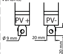
Obr. 10: Anschluss an S-Variante
