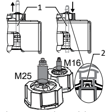
Şek. 14: EMC rakorundaki ekranlama yuvası
