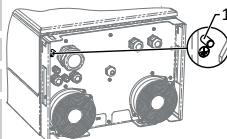
Imm. 12: Ulteriore punto di messa a terra
