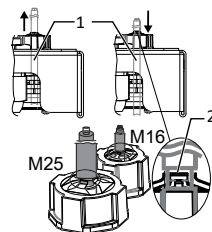
Afb. 14: Afschermingssteun op de EMC-schroefverbinding
