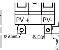
Rys. 9: Przyłącze do wariantu Basic+M
