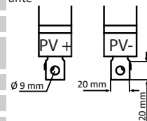
Áb. 10: Csatlakozás S-változatra
