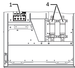
Afb. 6: Aansluitklemmen: S-versie
