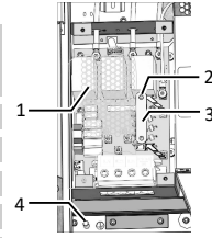
Áb. 3: 5-vezetékcsatlakozás
