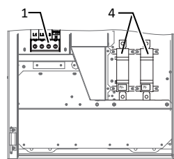
Fig. 6: Terminais de ligação: versão S
