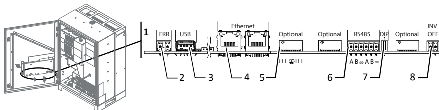
Fig. 13: Kommunikasjonsskort: Tilkobling og tildeling av grensesnittene
