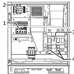
Fig. 5: Bornes de conexión versión M
