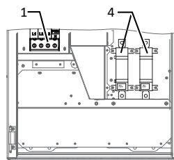
Fig. 6: Anslutningsklämmor: S-version
