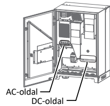
Áb. 7: Csatlakozókapsok
