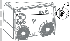
Afb. 12: Extra aardingspunt
