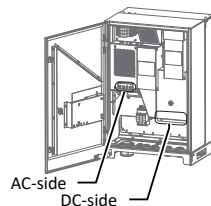
Fig. 7: Tilkoblingsklemmer
