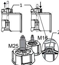
איור 14: מגן בחיבור הברגה EMC
