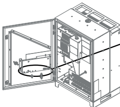
Fig. 13: Πλακέτα επικοινωνίας: Σύνδεση και αντιστοίχιση των θυρών
