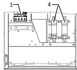
Fig. 6: Bornes de conexión: versión S
