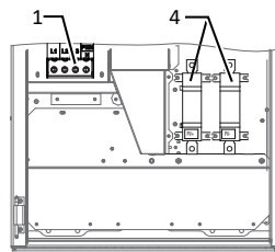
Fig. 6: Tilkoblingsklemmer: S-versjon
