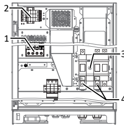
Áb. 5: Csatlakozókapsok M változathoz
