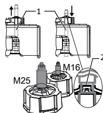
Áb. 14: Az EMC csavarkötés árnyékolóráté
