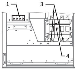
Áb. 4: Csatlakozókapsok - Basic változat
