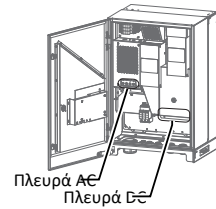
Fig. 7: Ακροδέκτες σύνδεσης
