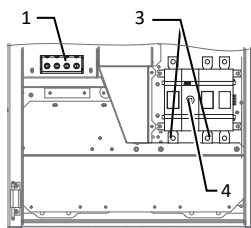
Fig. 4: Tilslutningsklemmer - Basic-ver-
