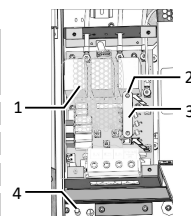
Fig. 3: 5-ledertilslutning
