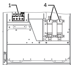
Fig. 6: Tilslutningsklemmer: S-version
