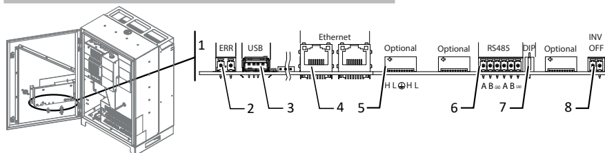
Imm. 13: Scheda di comunicazione: Collegamento e assegnazione delle interfacce
