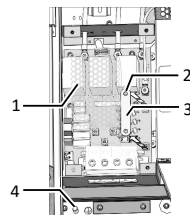
Fig. 3: 5-leders-tilkobling
