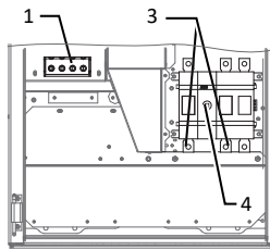
Fig. 4: Bornes de conexión - Versión Basic
