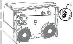
Abb. 12: Zusätzlicher Erdungspunkt
