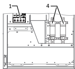
Sl. 6: Priključne sponke: različica S
