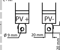
Rys. 10: Przyłącze do wariantu S
