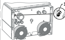
Fig. 12: Ponto de ligação à terra adicional
