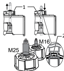
III. 14: Raccordement du blindage sur le vissage CEM
