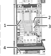
Şek. 3: 5 iletkenli bağlantı
