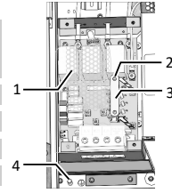
Kuva 3: 5-johdinliitäntä
