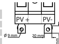
Fig. 9: Ligação à variante Basic+M
