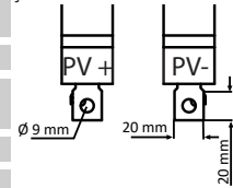
Şek. 10: S modeline bağlama
