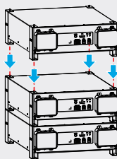
Método 1: Montado no piso
