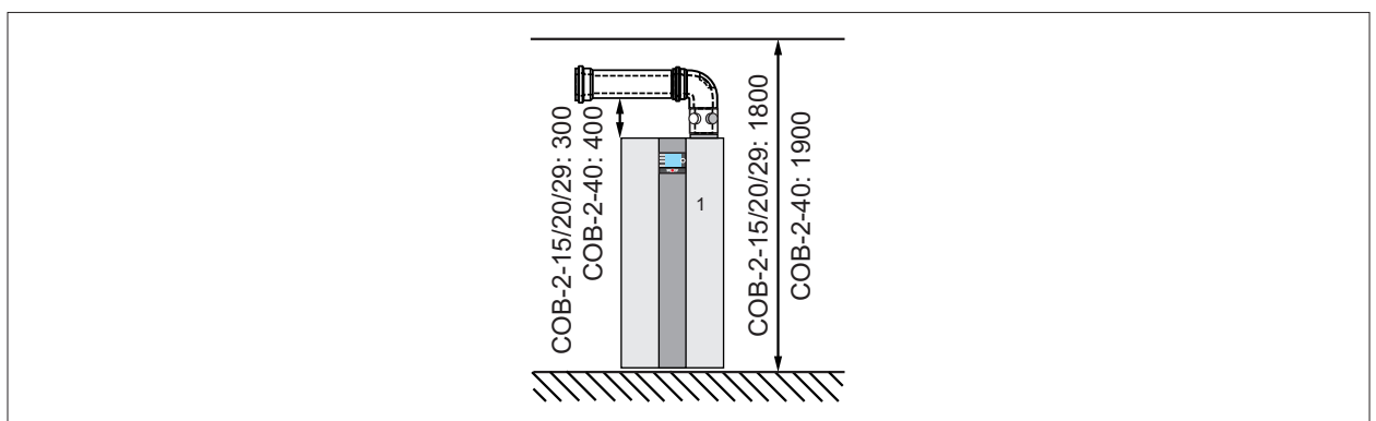
Afb. 4.2 Minimale afstanden omhoog [mm]
