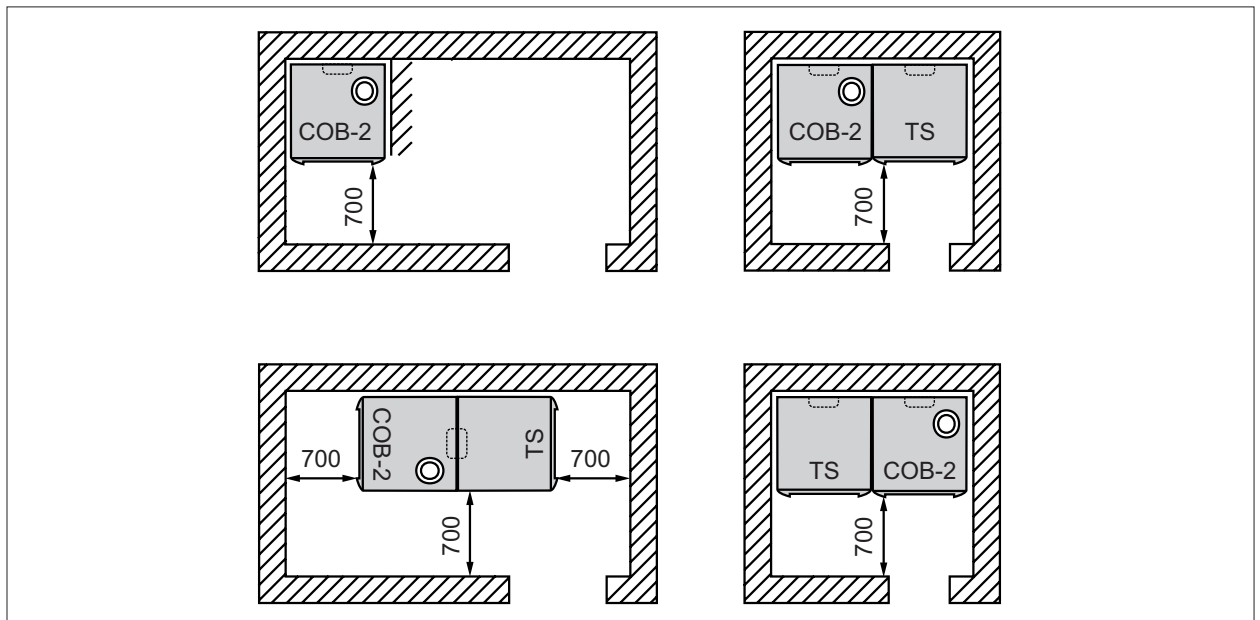
Afb. 4.1 Minimale wandafstanden [mm]
