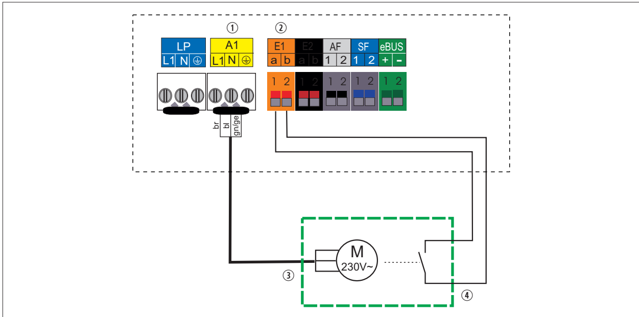
Afb. 12.3 Elektrische aansluiting HCM-2
