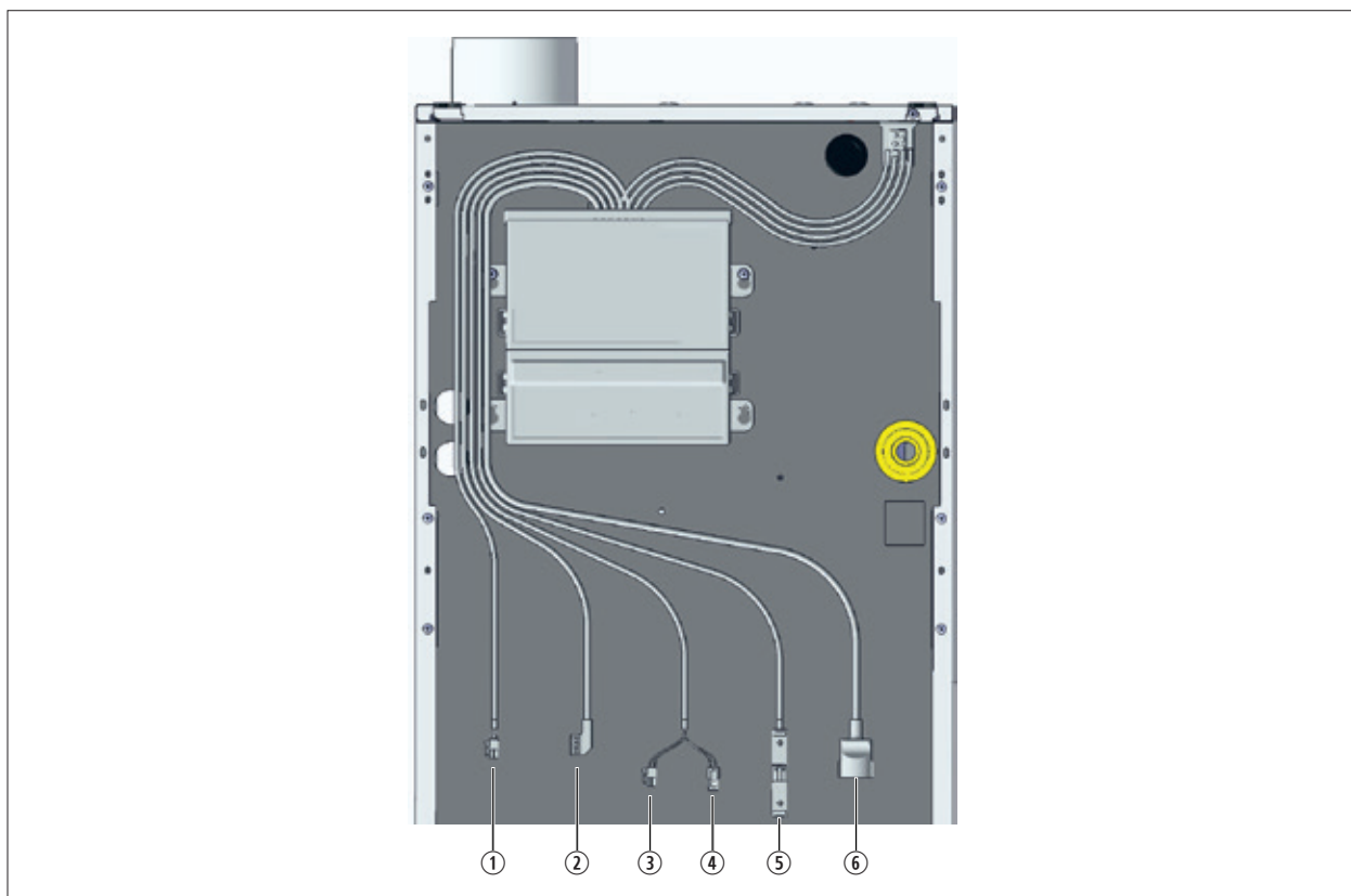
Afb. 5.21 Elektrische aansluiting aan de achterkant van de oliegestookte HR-ketel.
