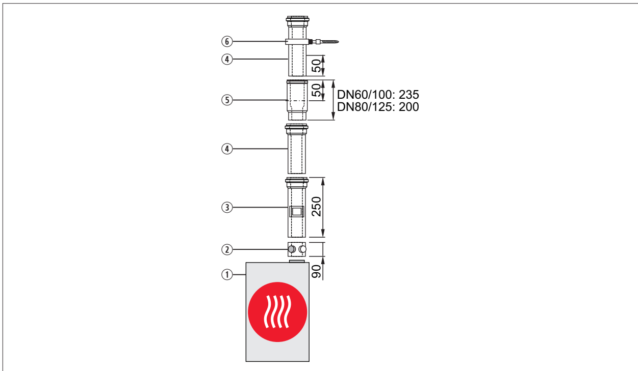
Afb. 5.14 Voorbeeld lucht-/rookgasgeleiding [mm]
