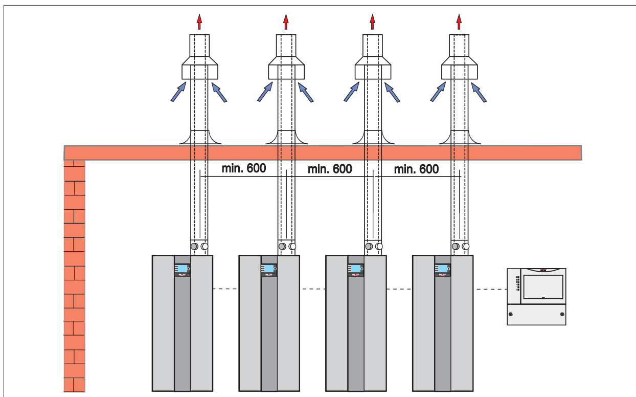
Afb. 4.9 Cascadesturing met gescheiden concentrische lucht-/rookgasgeleiding verticaal type C33x
