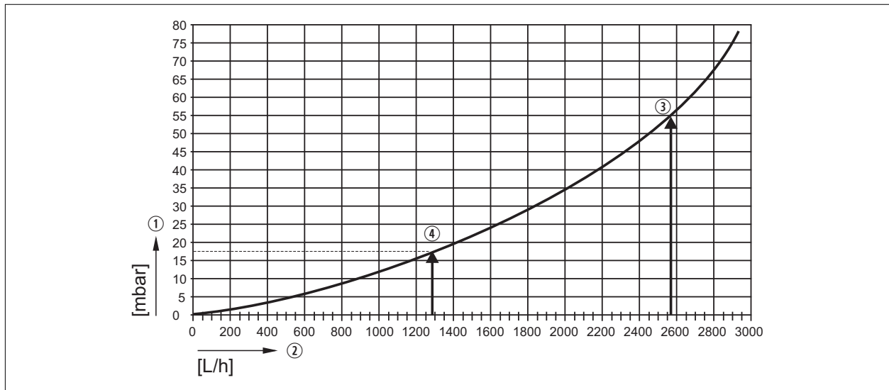
Afb. 11.7 Drukverlies bij verwarmingswater COB-2-29
