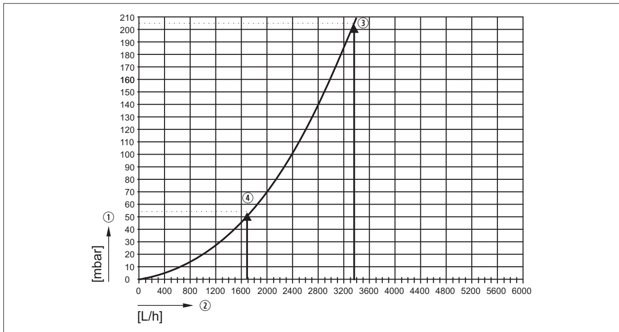
Afb. 11.8 Drukverlies bij verwarmingswater COB-2-40
