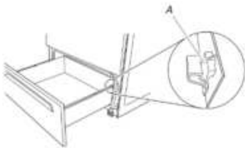
A. Glissière de tiroir engagée.
