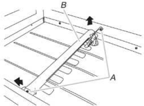
A. Tornillos B. Quemador para hornear
