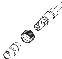
TA4F Gewindeadapter
