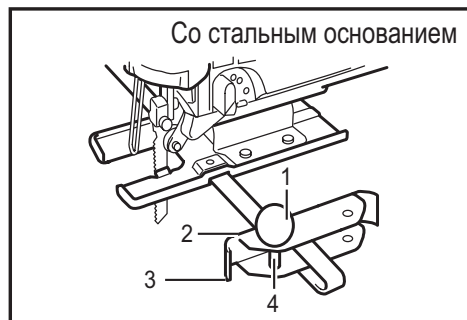
► Рис.22: 1. Резьбовая ручка 2. Направляющая смотрит 3. Направляющая планка (направляющая линейка) 4. Штифт
