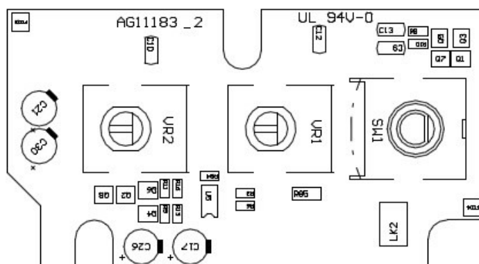
CUE B Assembly 004-988 (PCB AG11183)
