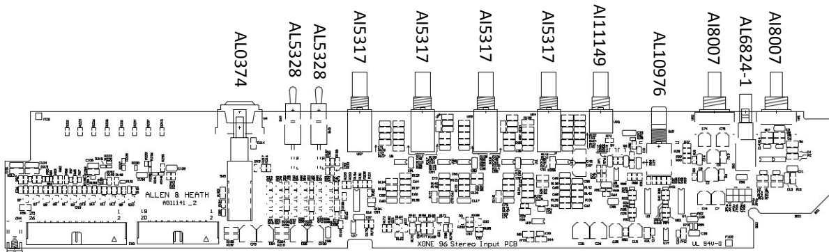
STEREO INPUT Assembly 004-966 (PCB AG11141)
