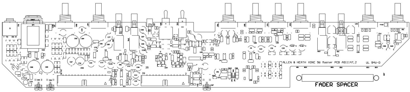
MASTER Assembly 004-972 (PCB AG11147)
