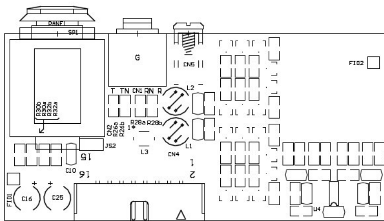
CUE B Assembly 004-988 (PCB AG11183)
