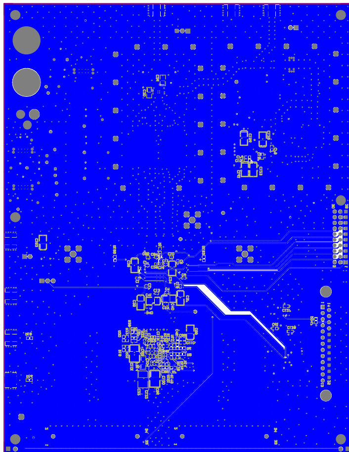
Figure 20. Bottom Layer
