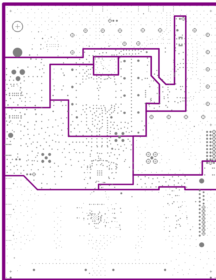
Figure 19. Layer 5
