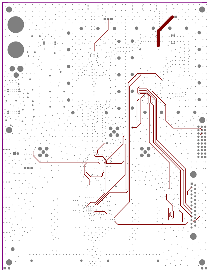
Figure 18. Layer 4 (NH)
