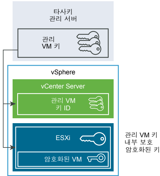
그림 6-2. vSphere 가상 암호화 아키텍처
