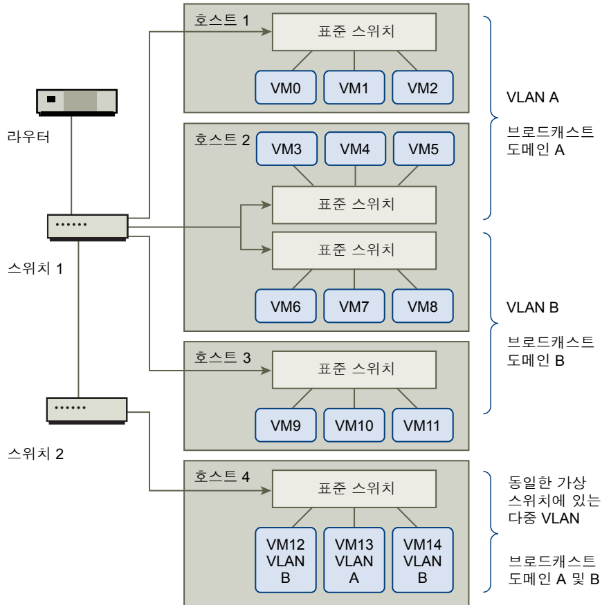
그림 10-1. 샘플 VLAN 레이아웃
