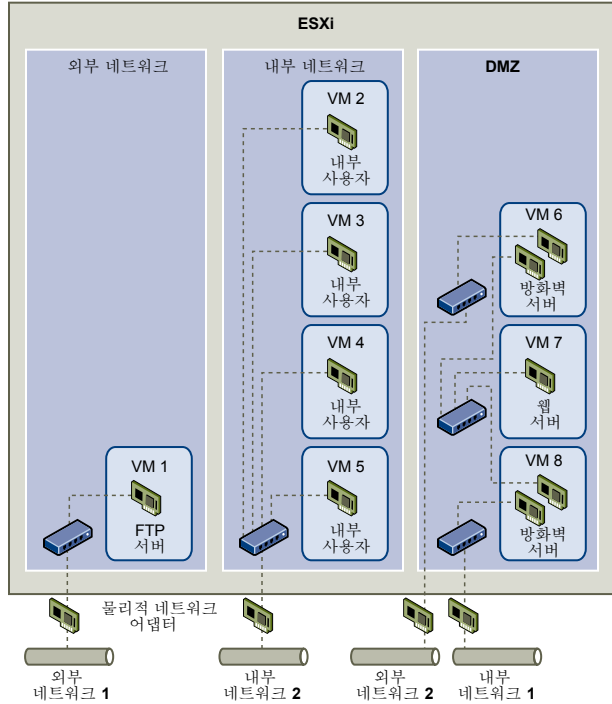
그림 10-2. 단일 ESXi 호스트에 외부 네트워크, 내부 네트워크 및 DMZ 구성
