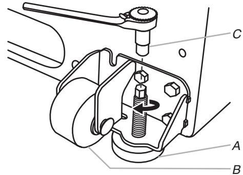
A. Pata de freno B. Rodillo frontal C. Destornillador hexagonal de 1/4"
