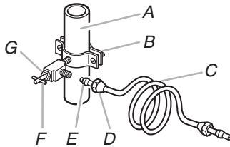
A. Tubería de agua fría B. Abrazadera para tubería C. Tubería de plástico D. Tuerca de compresión E. Manga de compresión F. Válvula de cierre G. Tuerca de presión
