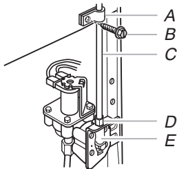
A. Abrazadera para tubería B. Tornillo de la abrazadera para tubería C. Tubería de plástico D. Tuerca de compresión E. Entrada de la válvula
