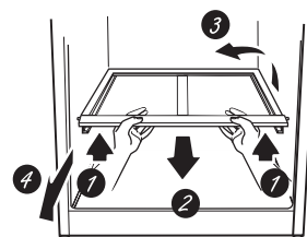
Pour enlever le cadre
