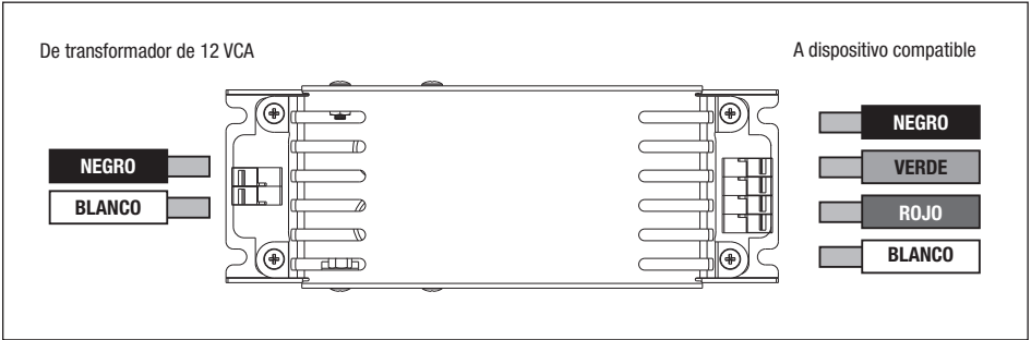
Figura 5. Cableado RGB
