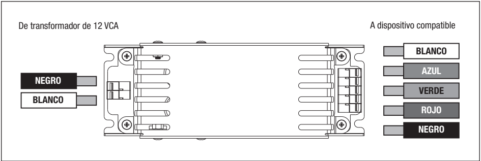
Figura 6. Cableado RGBW
