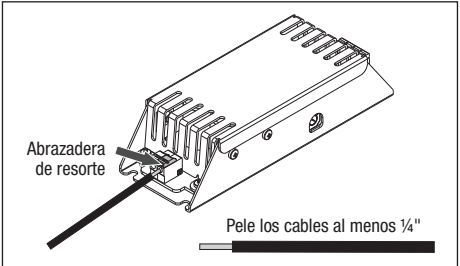
Figura 4. Pelar e insertar los cables
