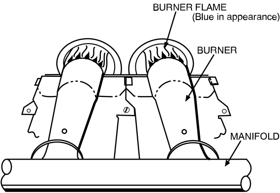
Fig. 15 – Monoport Burner
