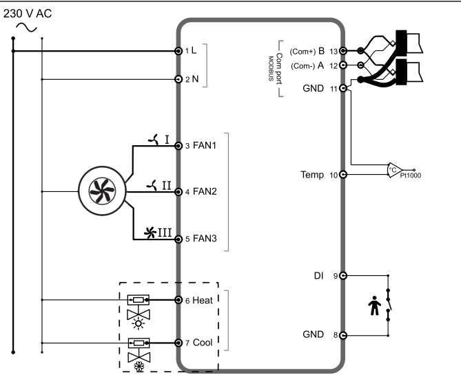
Bild 1 4-Rohr-Verdrahtung
