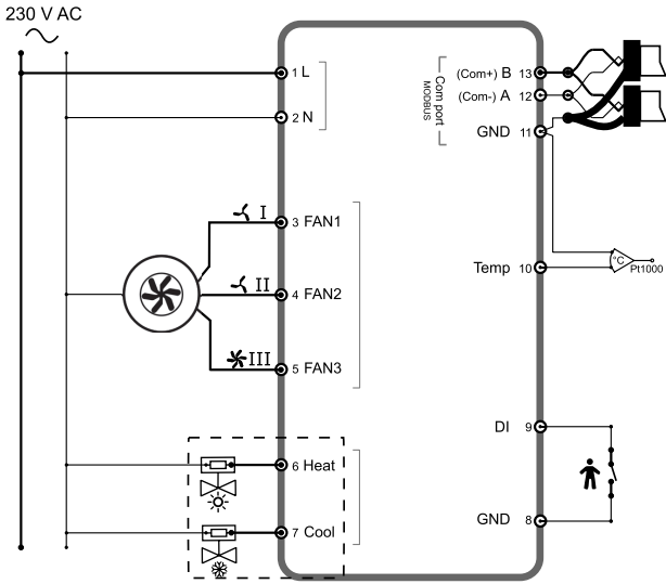
Fig. 1 Raccordement à 4 tubes
