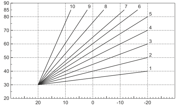
şek. 11 - Kompensasyon eğrisi
