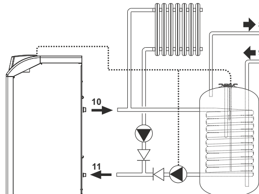
мал. 14 - Схема під'єднання до зовнішнього бойлера
