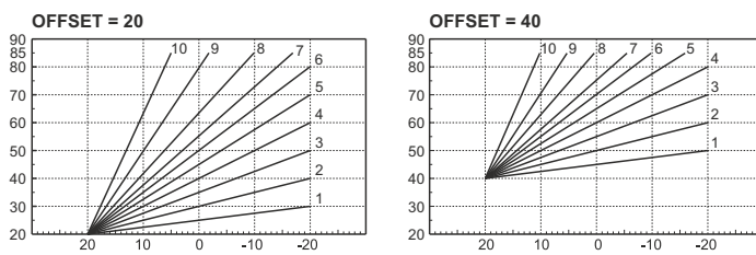
мал. 12 - Пиклад паралельного пересування компенсаційних кривих
