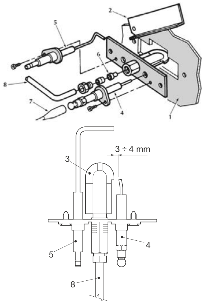
fig. 21 - Brûleur pilote
