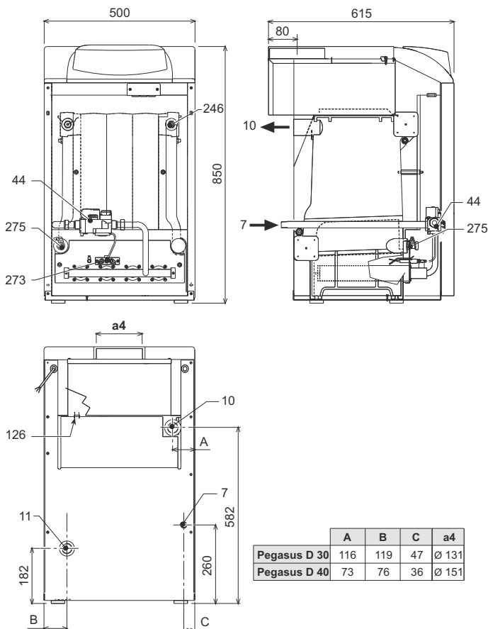
sek. 23 - Boyutlar ve eklentiler mod. PEGASUS D 32 e PEGASUS D 45
