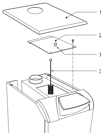
рис. 19 - Очистка котла
