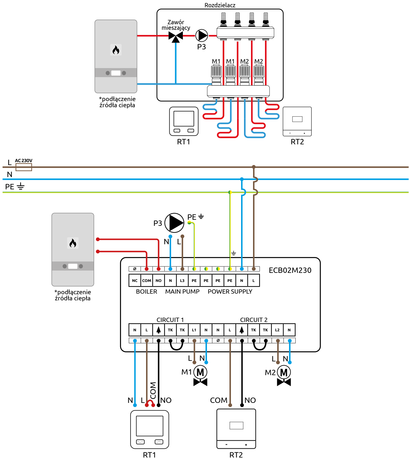
b) - Podłączenie 2 stref grzewczych ogrzewania podłogowego
