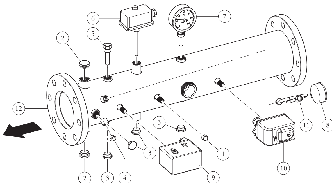
Installazione con connessione idraulica a sinistra / Installation with hydraulic connection on the left
