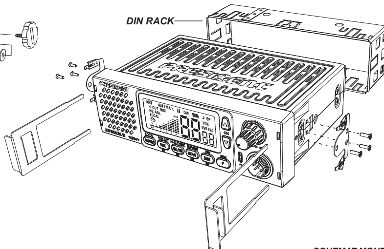
SCHEMAT MONTAŻU
