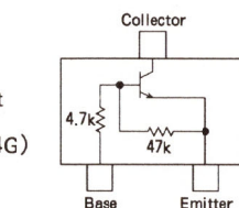
DTC143ZE (E23) (Q1009, 1026)
