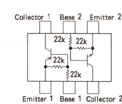
XP4312 (7T) (Q1017, 1025)
