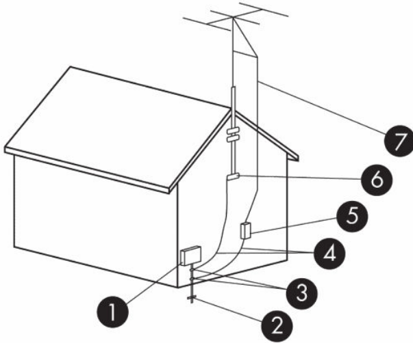
جدول ٣-٢ تأريض الهوائي
