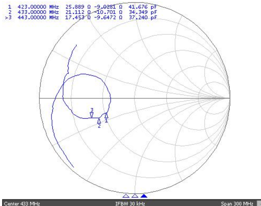
史密斯圆图 (Smith chart)
