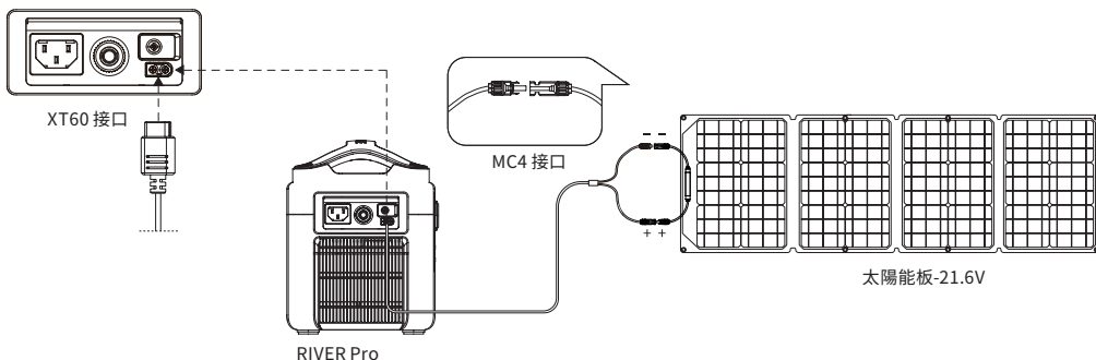
RIVER Pro充電接口區域
