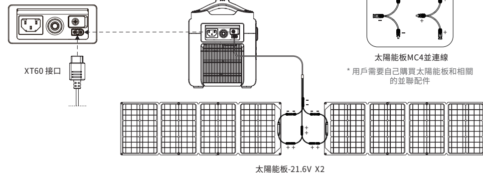
RIVER Pro充電接口區域
