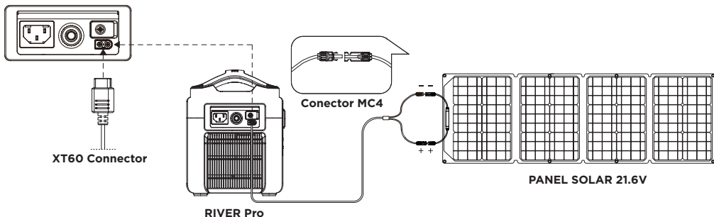
Puerto de Carga RIVER Pro
