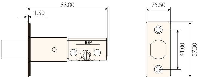
سقاطة قفل مركب (الوحدة: مم)
